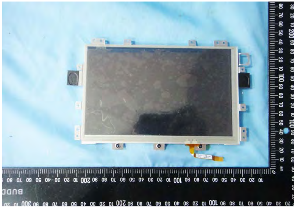
EUT Photo 42 )
