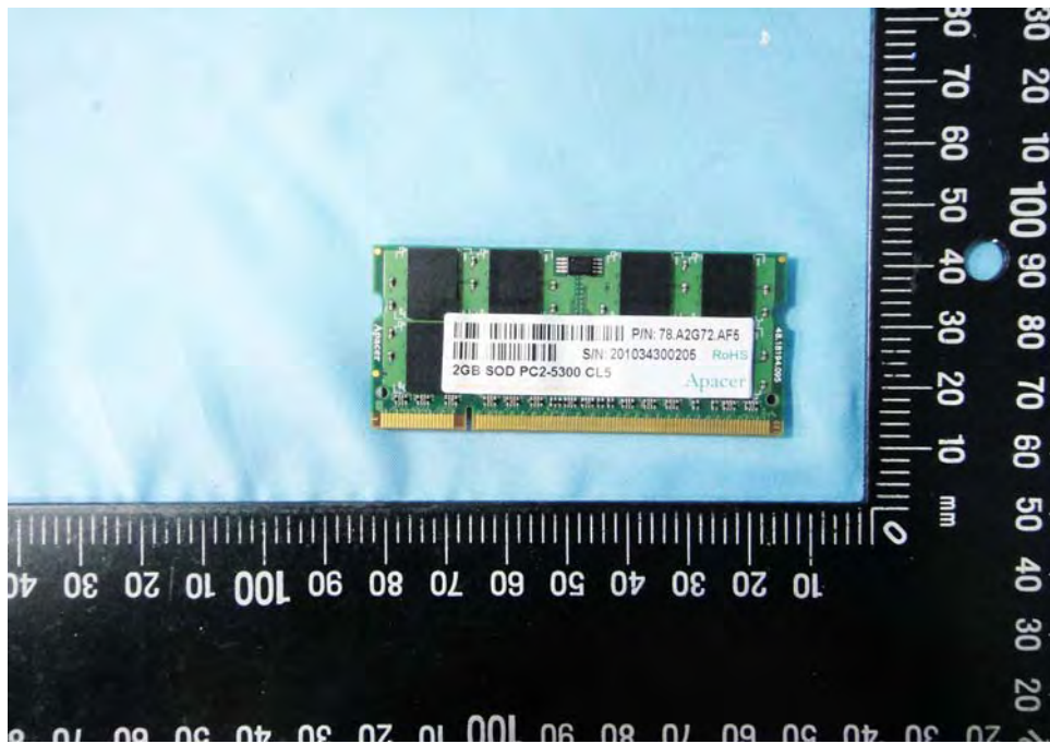
EUT Photo 28 )
