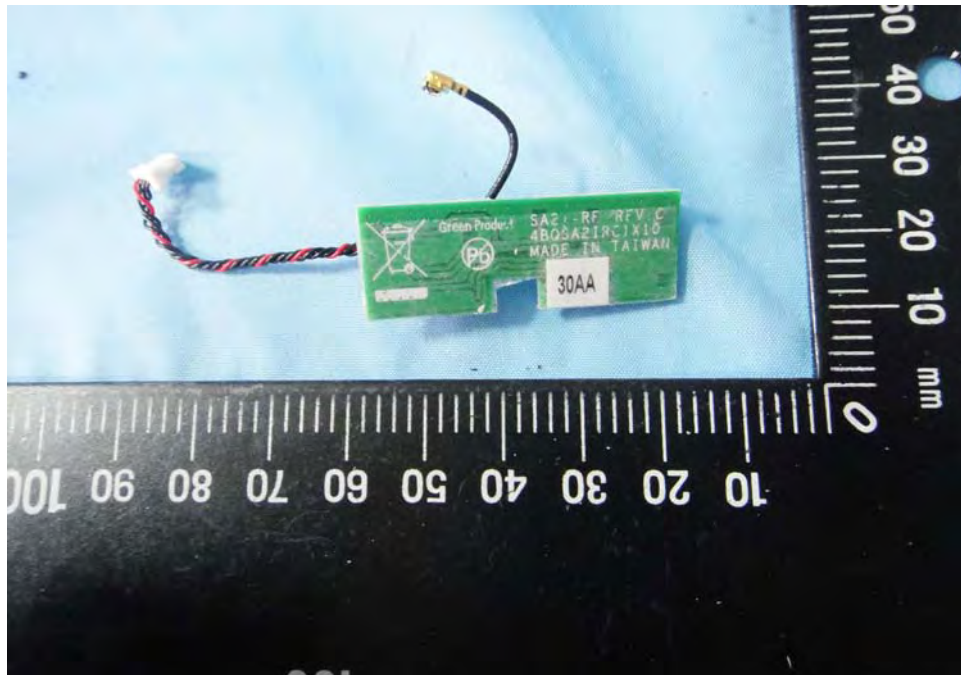
EUT Photo 48 )
