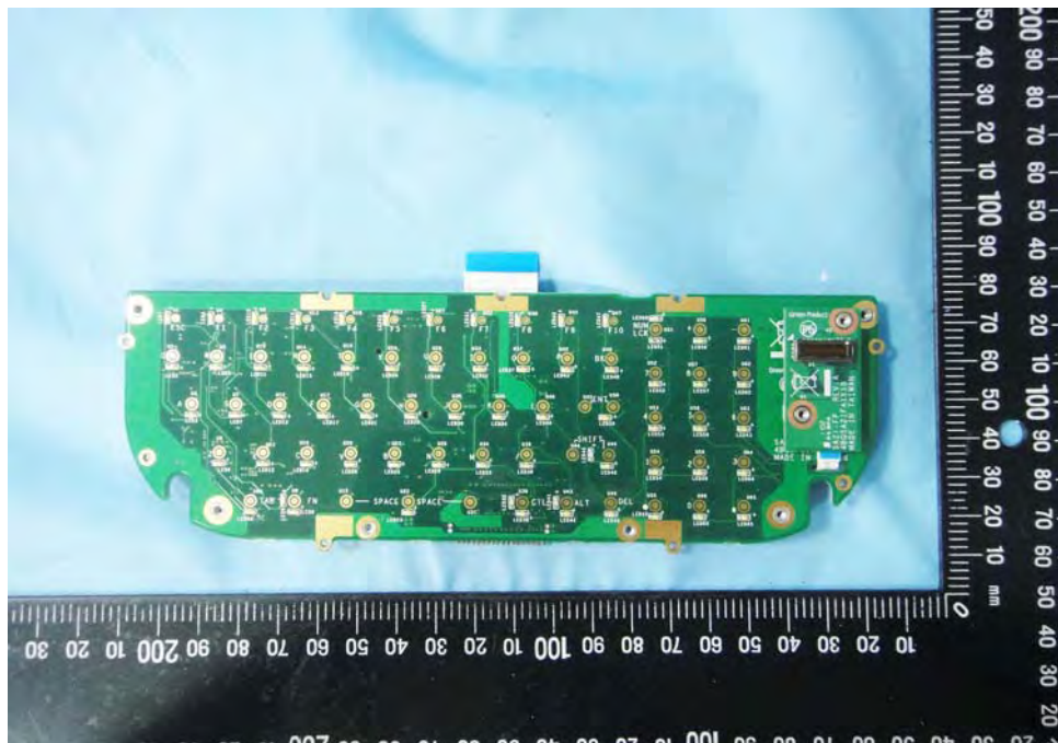
EUT Photo 46 )
