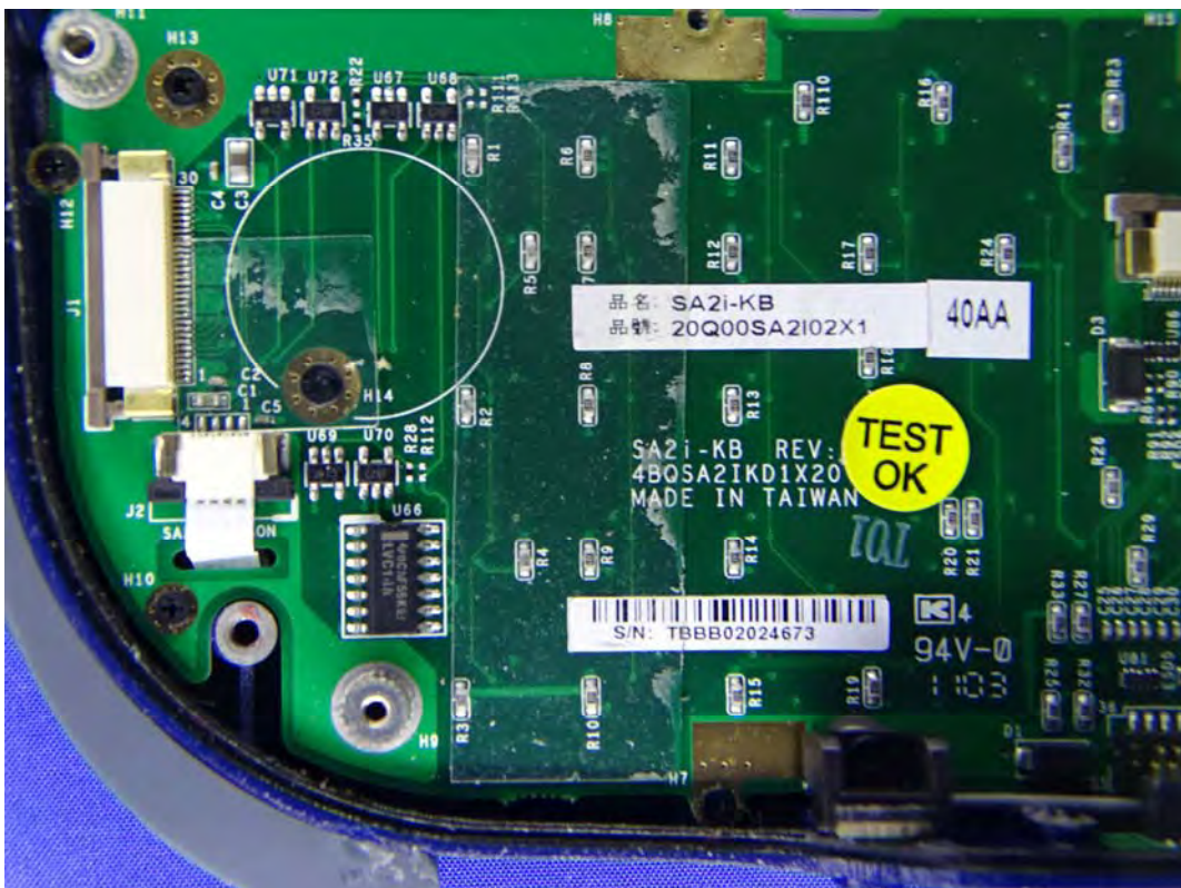
(93) EUT Photo
