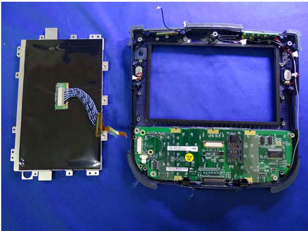
(83) EUT Photo
