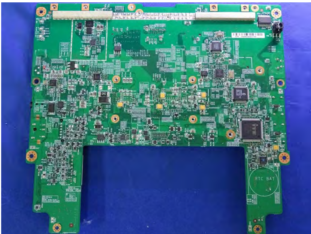
(75) EUT Photo
