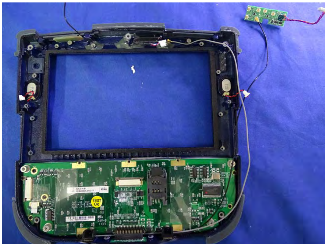
(95) EUT Photo
