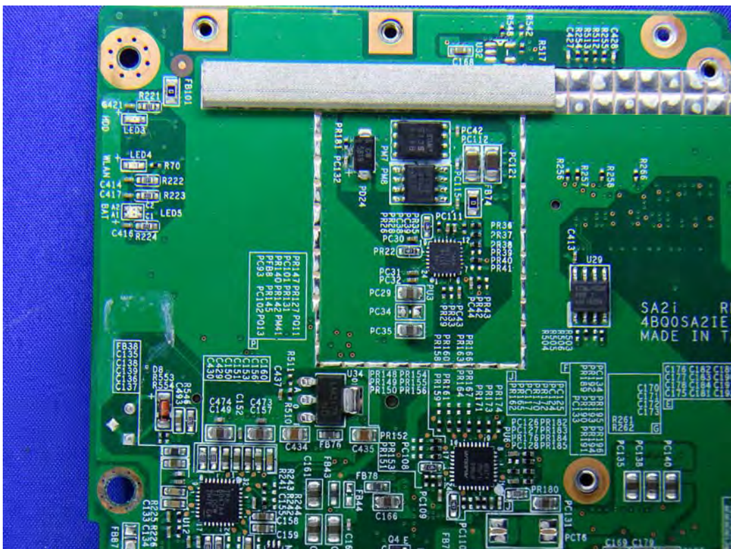
(65) EUT Photo
