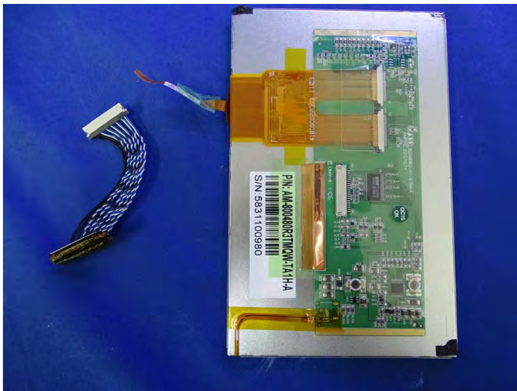
(88) EUT Photo
