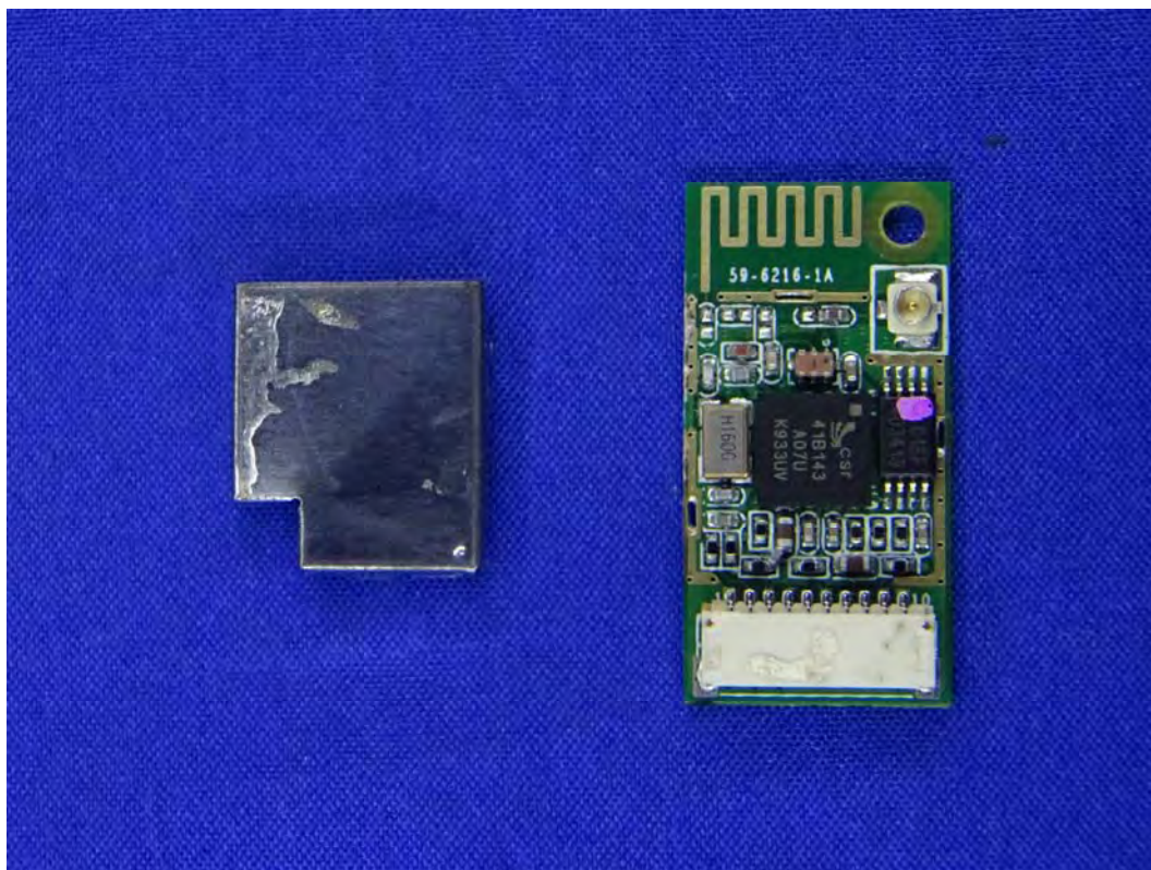
(60) EUT Photo
