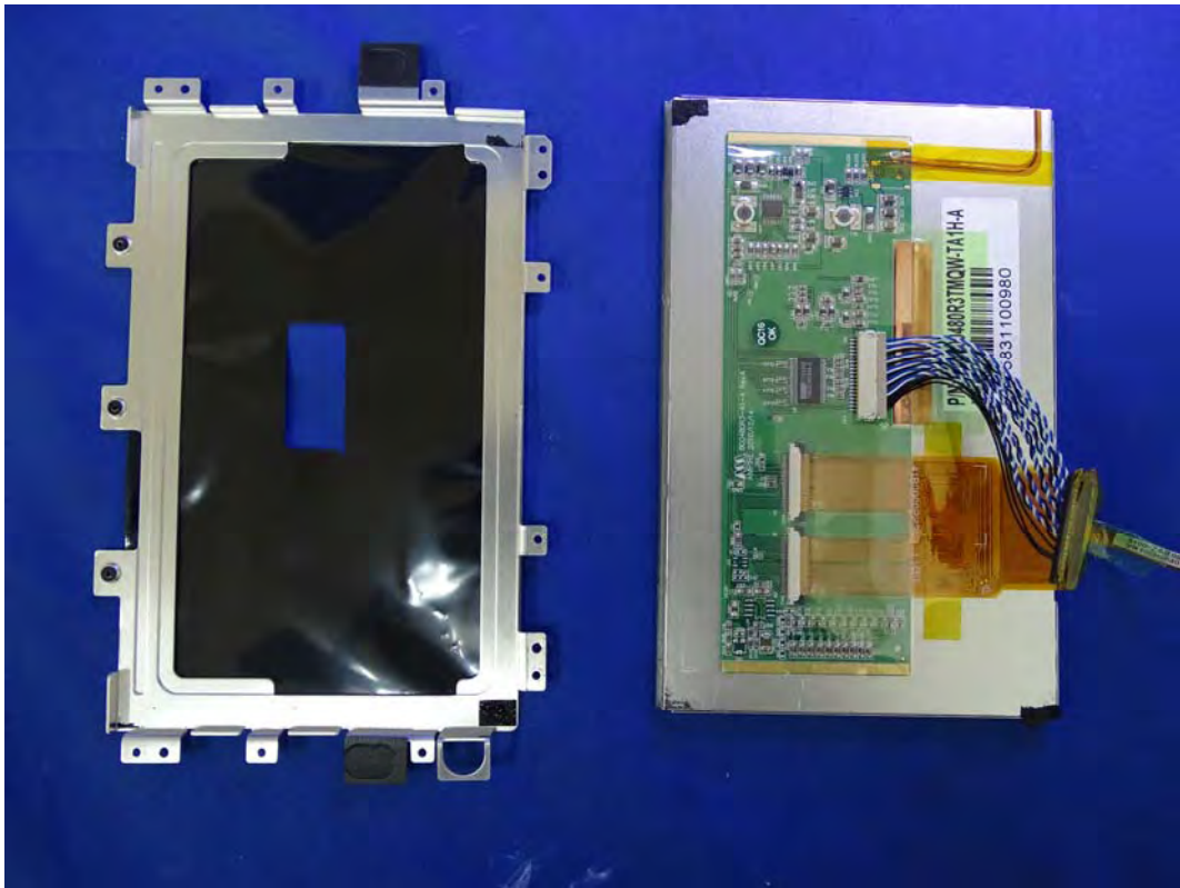
(86) EUT Photo
