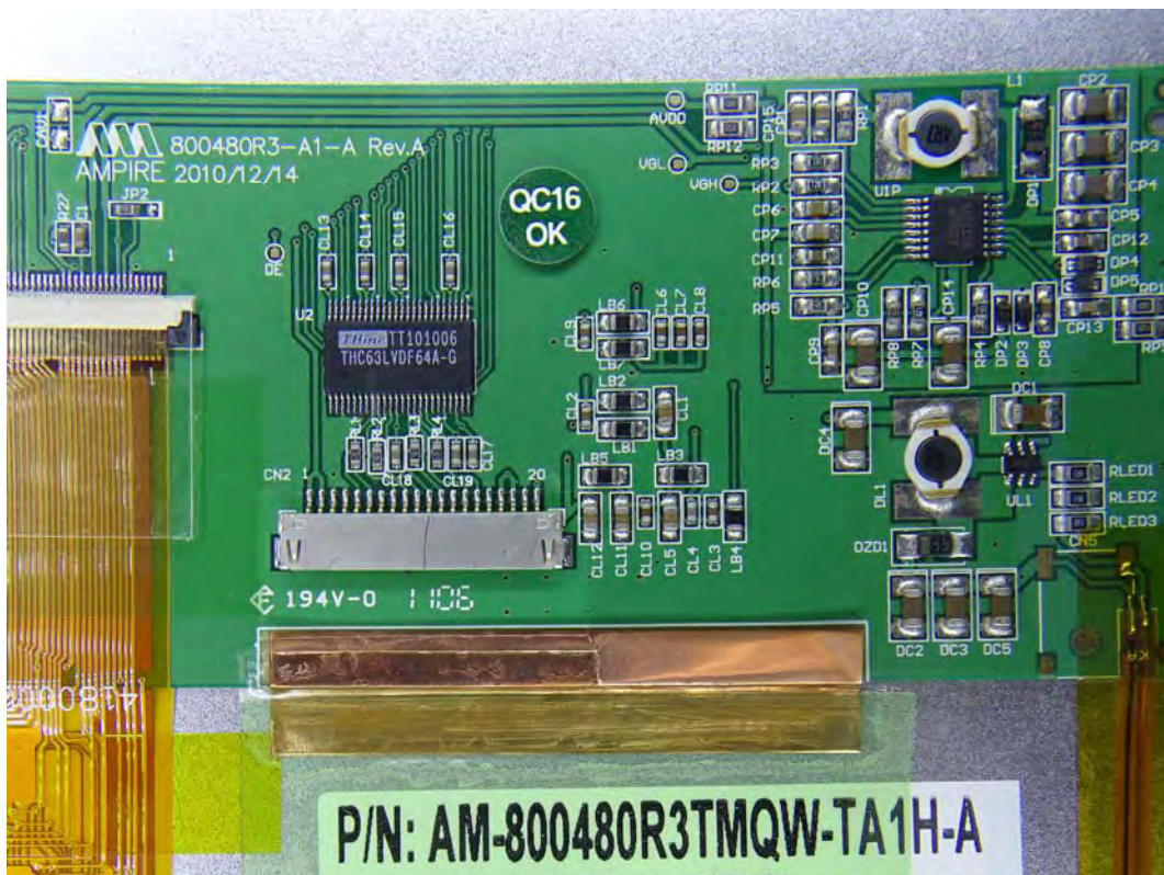
(91) EUT Photo
