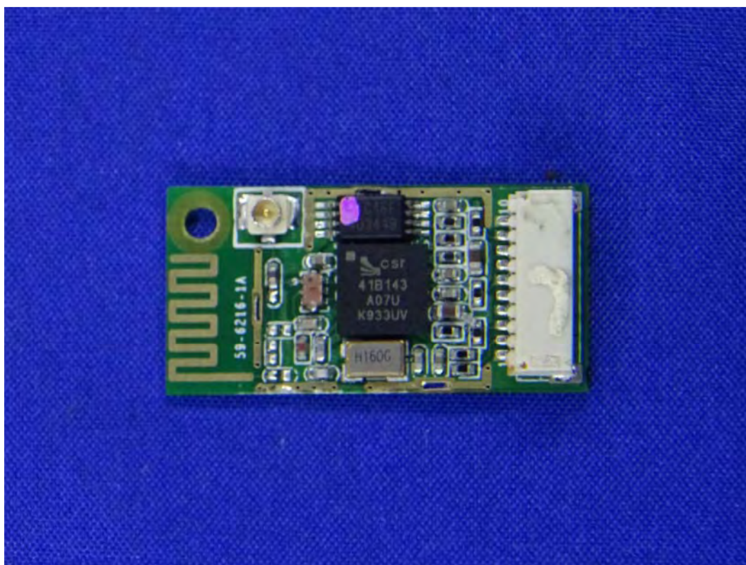
(61) EUT Photo
