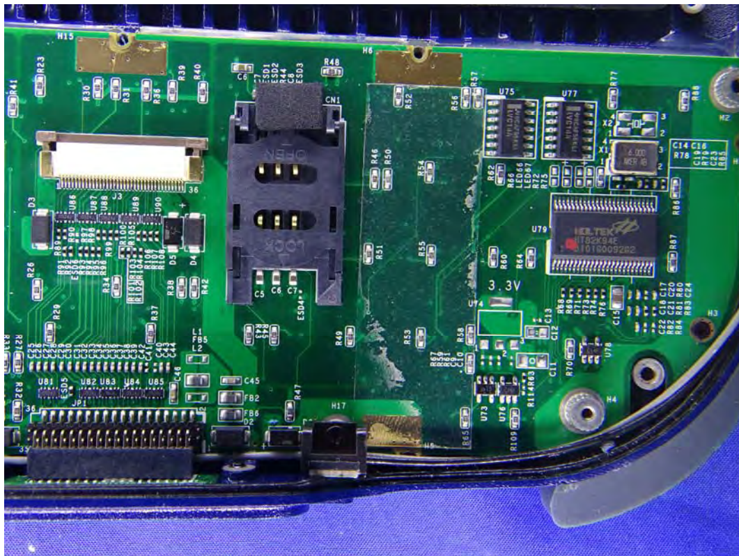
(94) EUT Photo
