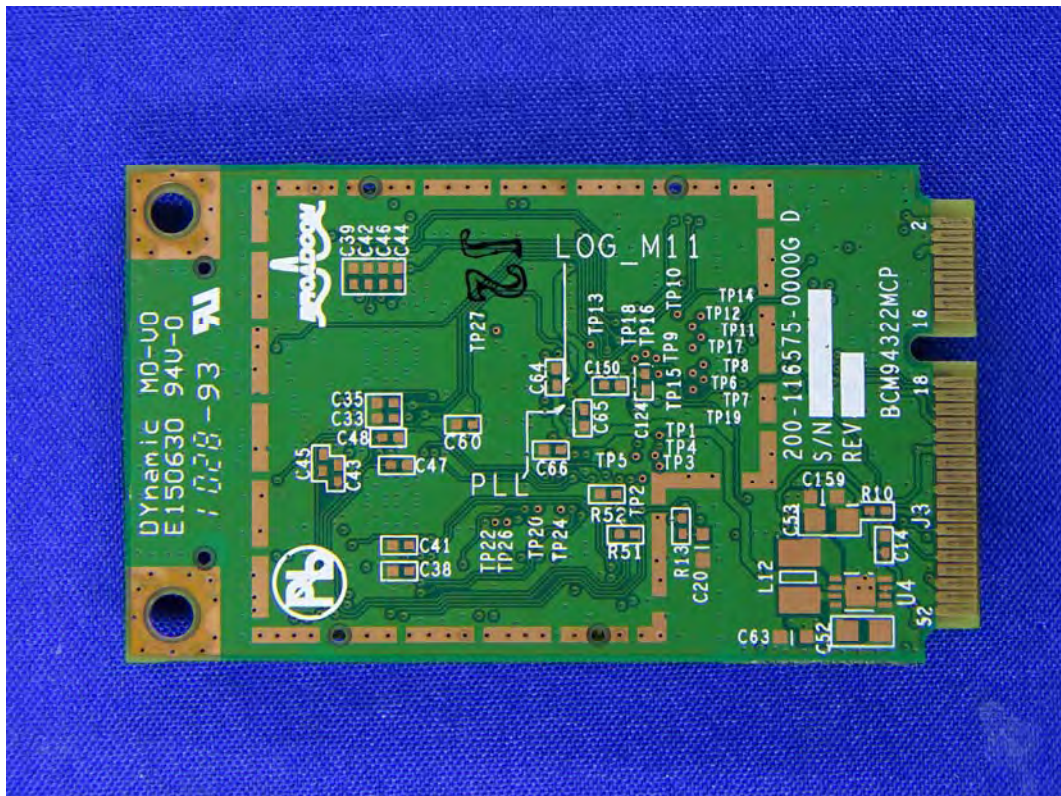
(25) EUT Photo-RF Module
