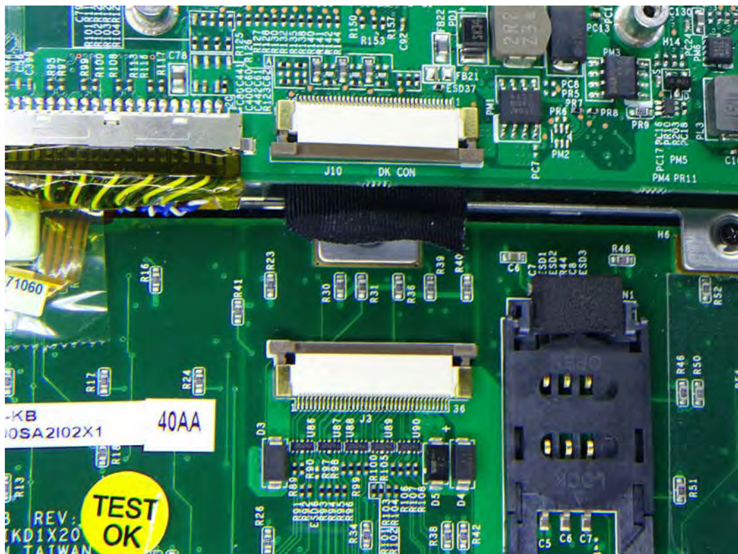
(50) EUT Photo
