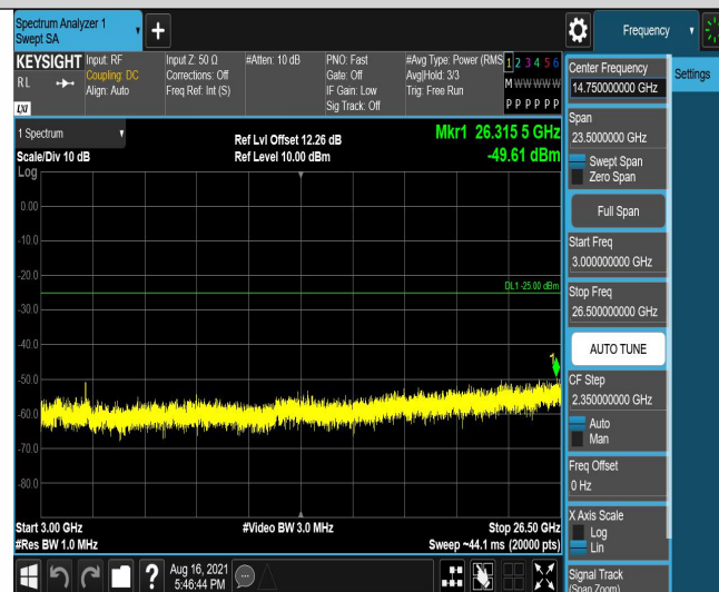
Band7-10MHz-QPSK-20800-50RB#0-Range3:3000~26500MHz
