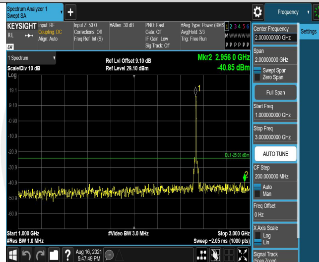
Band7-10MHz-QPSK-21100-50RB#0-Range2:1000~3000MHz
