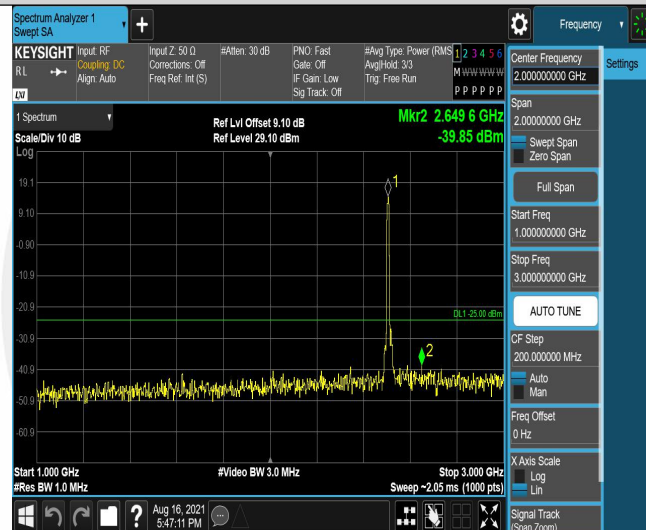
Band7-10MHz-16QAM-20800-50RB#0-Range2:1000~3000MHz
