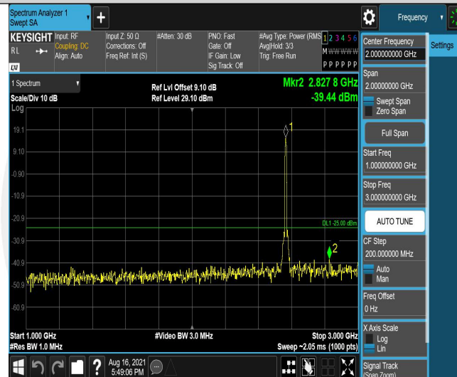
Band7-10MHz-QPSK-21400-50RB#0-Range2:1000~3000MHz
