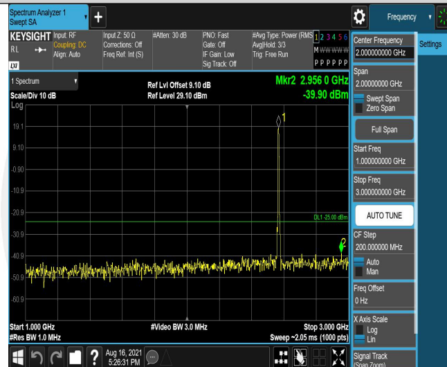
Band7-5MHz-QPSK-21425-25RB#0-Range2:1000~3000MHz
