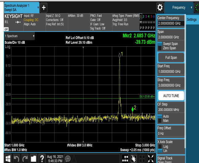
Band7-10MHz-QPSK-20800-50RB#0-Range2:1000~3000MHz
