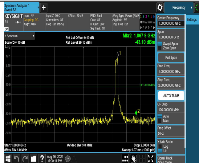
Band4-20MHz-QPSK-20175-100RB#0-Range2:1000~2000MHz
