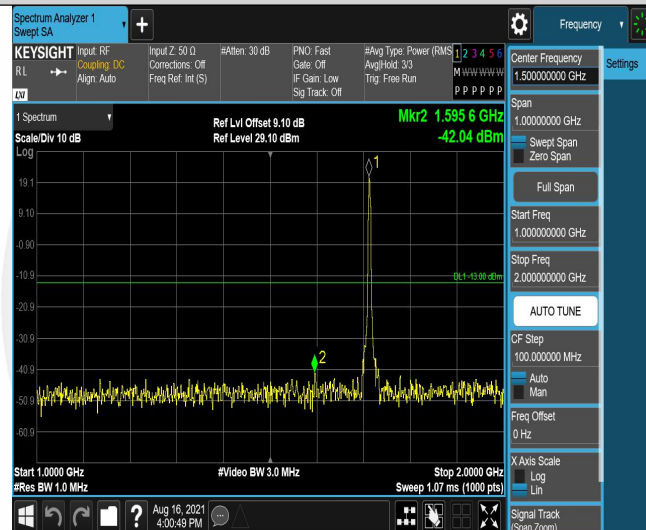
Band4-5MHz-QPSK-19975-25RB#0-Range2:1000~2000MHz
