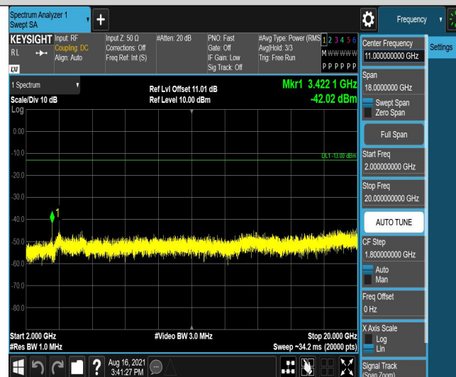
Band4-3MHz-QPSK-19965-6RB#0-Range3:2000~20000MHz
