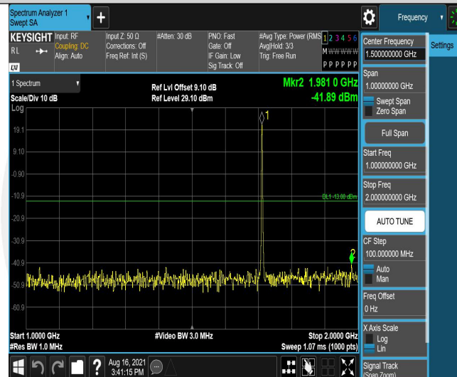
Band4-3MHz-QPSK-19965-6RB#0-Range2:1000~2000MHz
