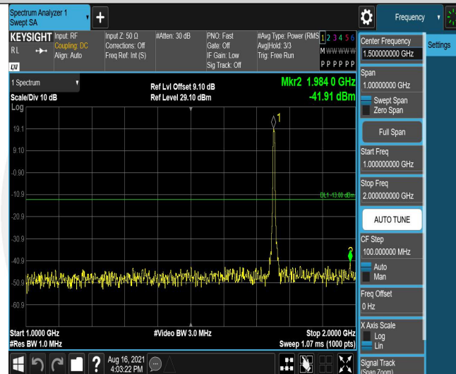
Band4-5MHz-QPSK-20375-25RB#0-Range2:1000~2000MHz
