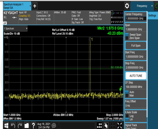
Band4-3MHz-16QAM-19965-6RB#0-Range2:1000~2000MHz
