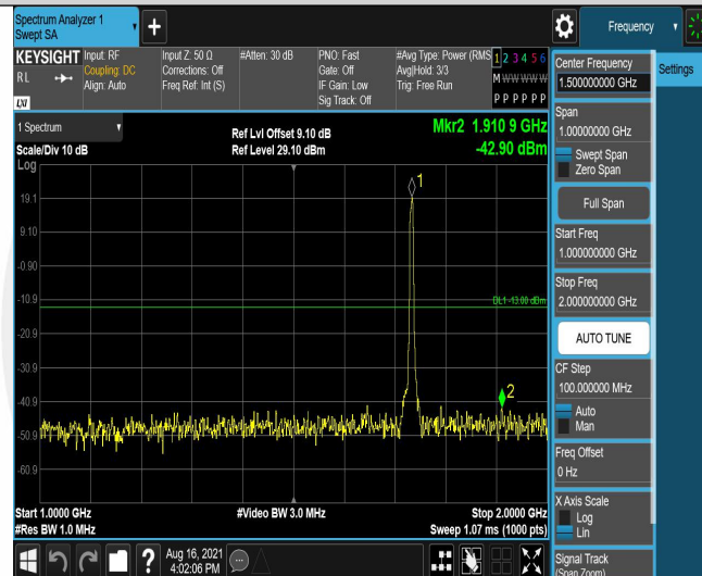
Band4-5MHz-QPSK-20175-25RB#0-Range2:1000~2000MHz
