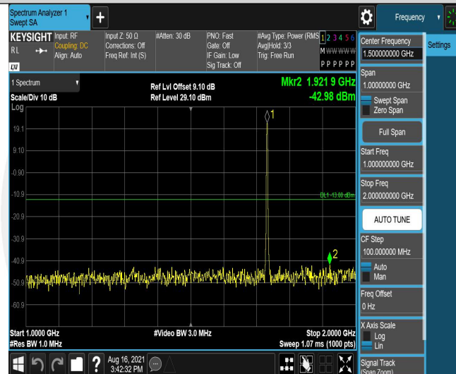
Band4-3MHz-QPSK-20175-6RB#0-Range2:1000~2000MHz
