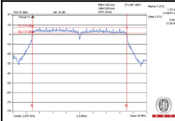
802.11n (20MHz)
