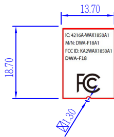
X-1850 下蓋銘版尺寸
