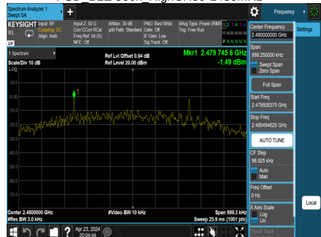
PSD BLE 500k HighCH39-2480MHz
