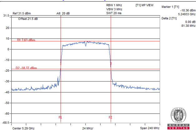
802.11ac (VHT80+80)_Chain 1 / CH58
