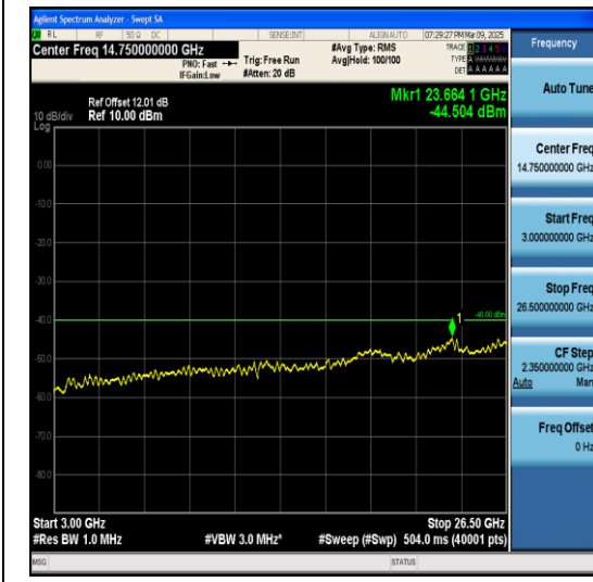
Band40(2345-2360)-10MHz-QPSK-39175-1RB#0-3000~26500-PASS
