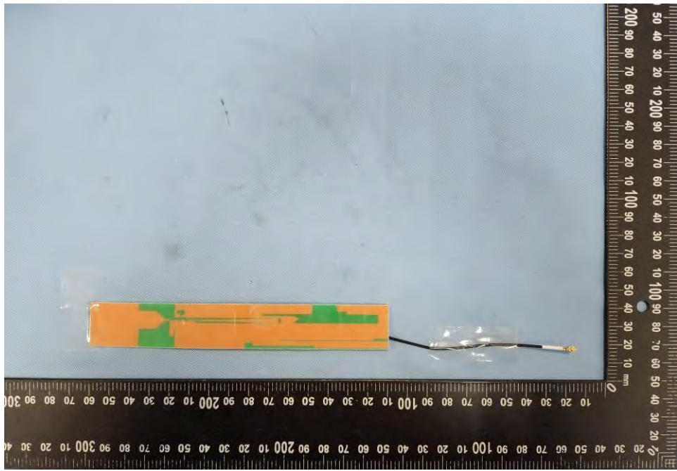
EUT Photo (44)
