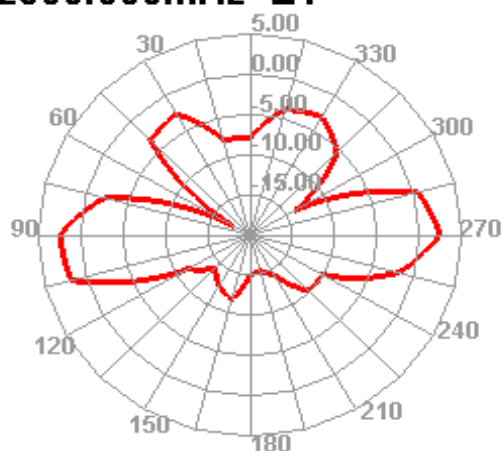
2500.000MHz E1
