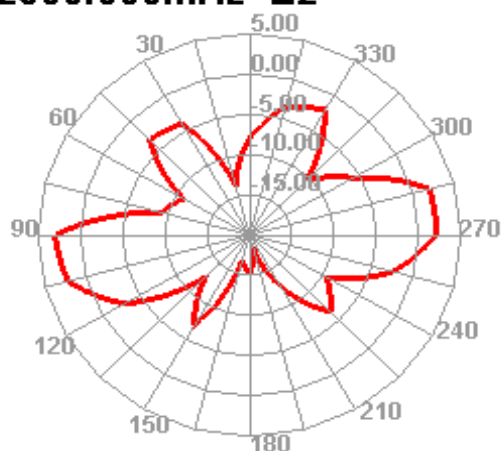
2500.000MHz E2
