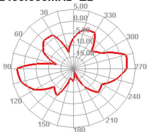
2450.000MHz E2
