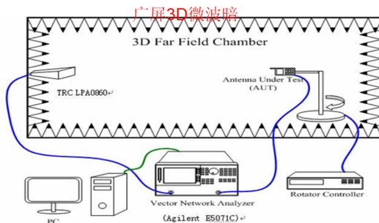
图. 1. 微波暗室内仪器设置 r.
