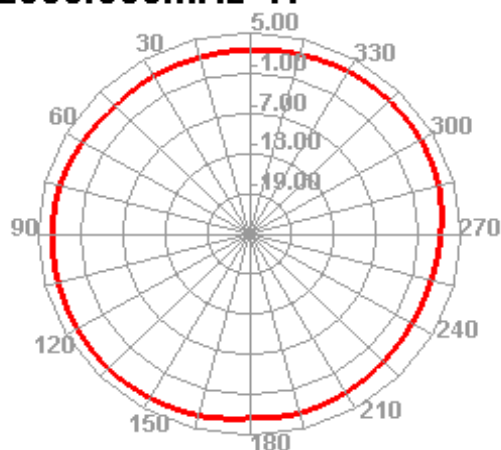
2500.000MHz H
