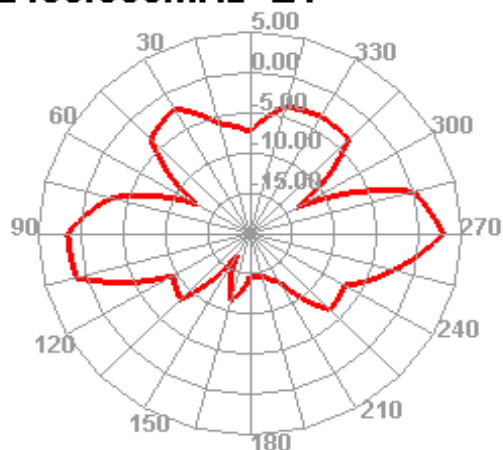
2450.000MHz E1
