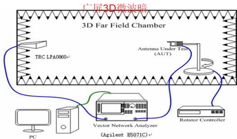
图. 1. 微波暗室内部仪器设置 r.
