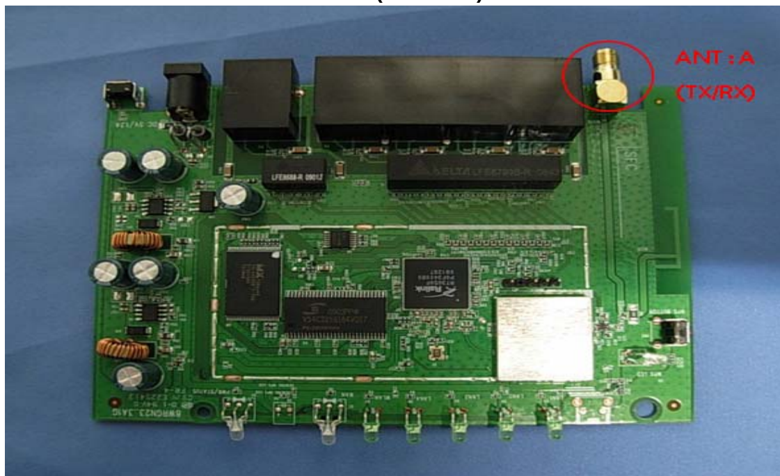
ANT A (1 TX/1 RX)
