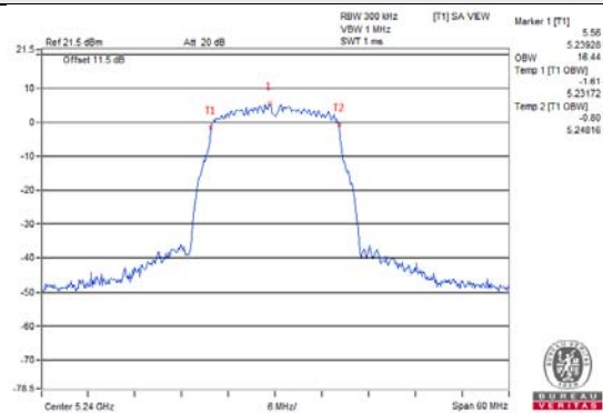
802.11a / Chain 1 / CH 48
