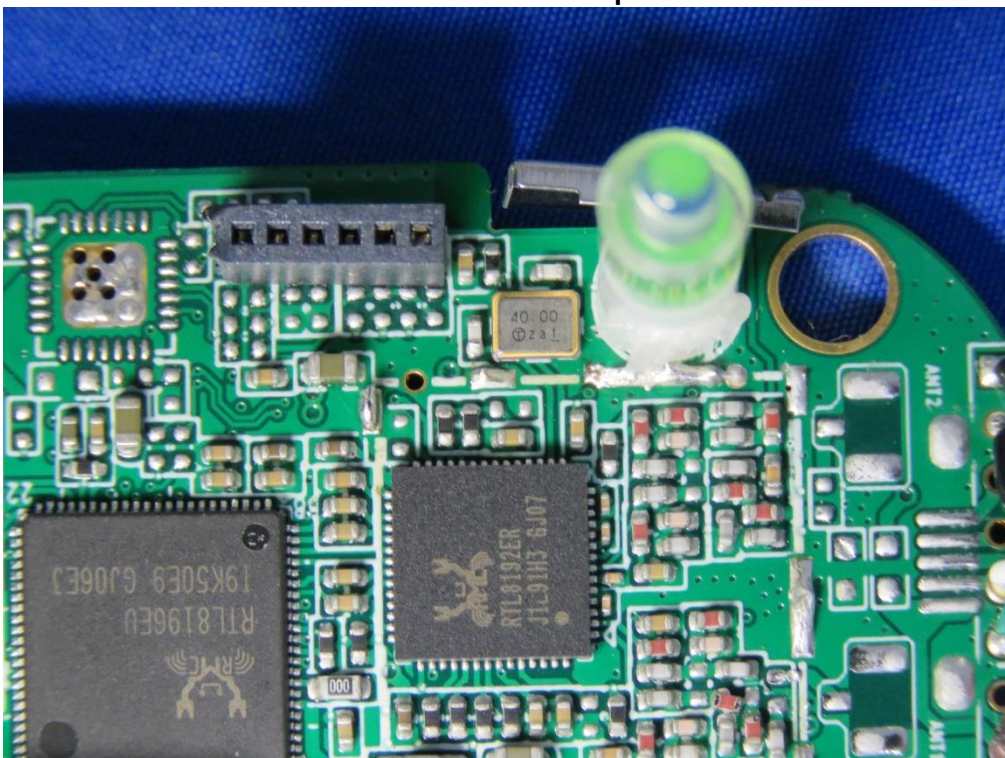
Wi-Fi Module Chip
