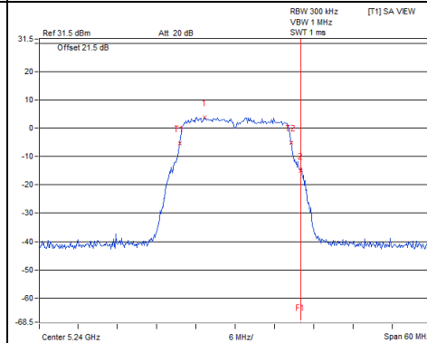
802.11a_Chain 3 / CH48
