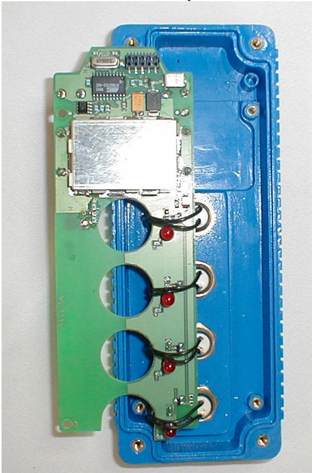
TP100 PCB Top
