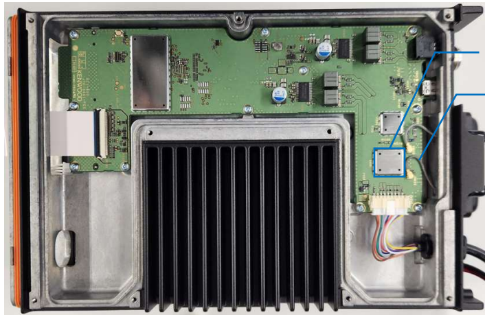
Bluetooth/WiFi Module
