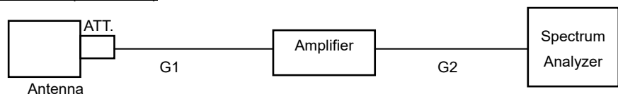
Above 1GHz(18-26.5GHz)
