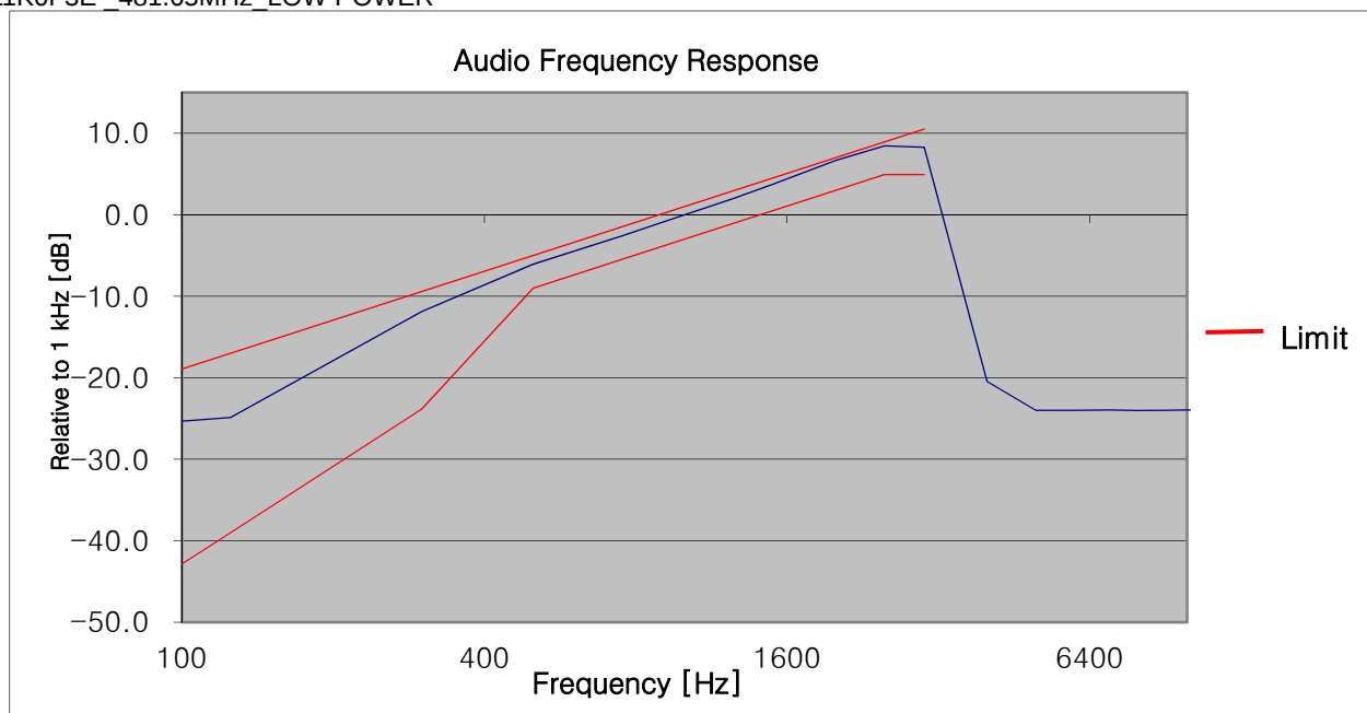
11K0F3E_481.05MHz_LOW POWER
