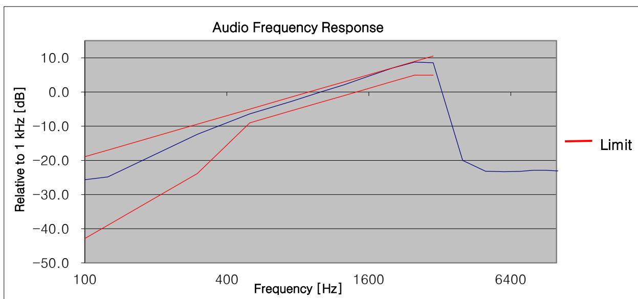
11K0F3E_150.05MHz_HIGH POWER
