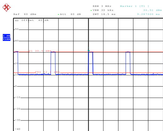
1880MHz - GSM
