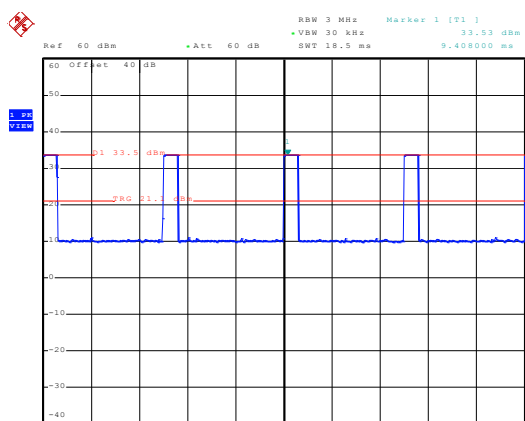
835MHz - GSM
