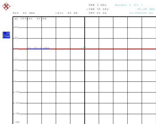
1880MHz - CW
