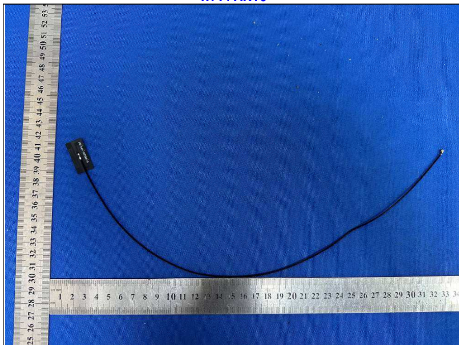
Wi-Fi ANT0
