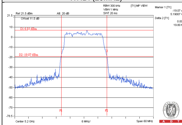
WHDI (20MHz)
