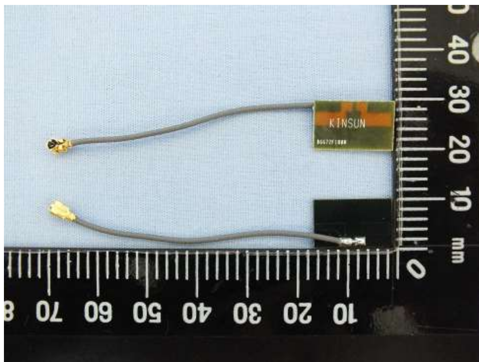
Antenna: 66722133B1-050
