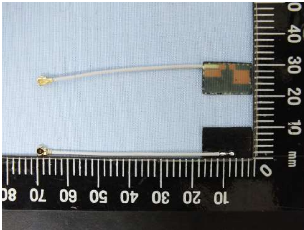
Antenna: F-F0010019-1
