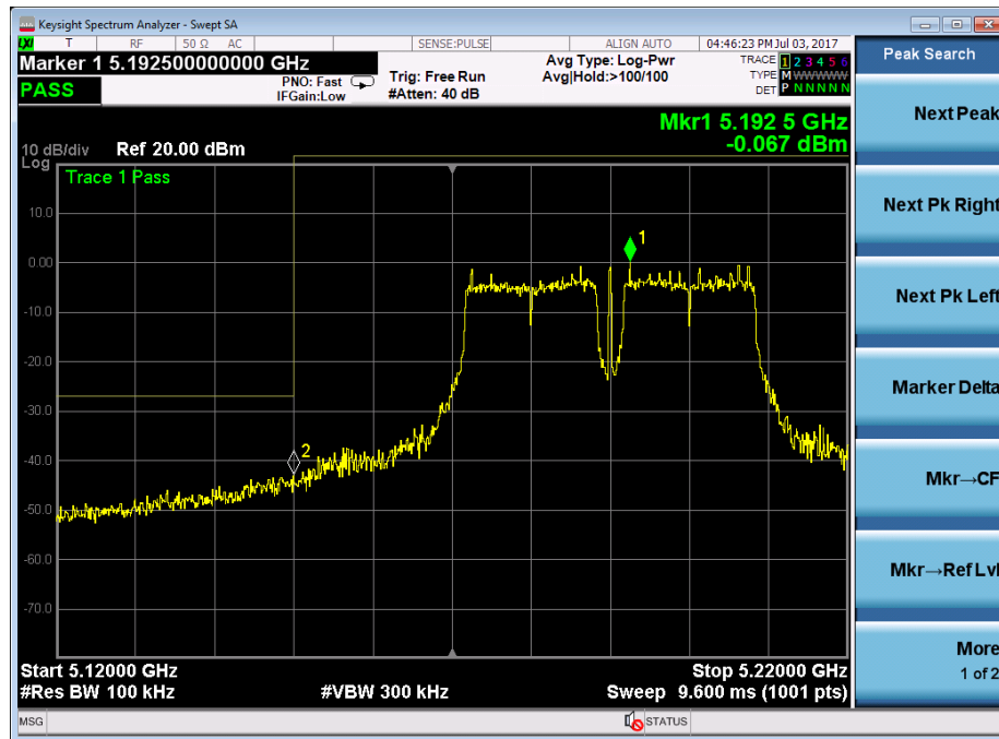
802.11ac(40): Band Edge, Left Side
