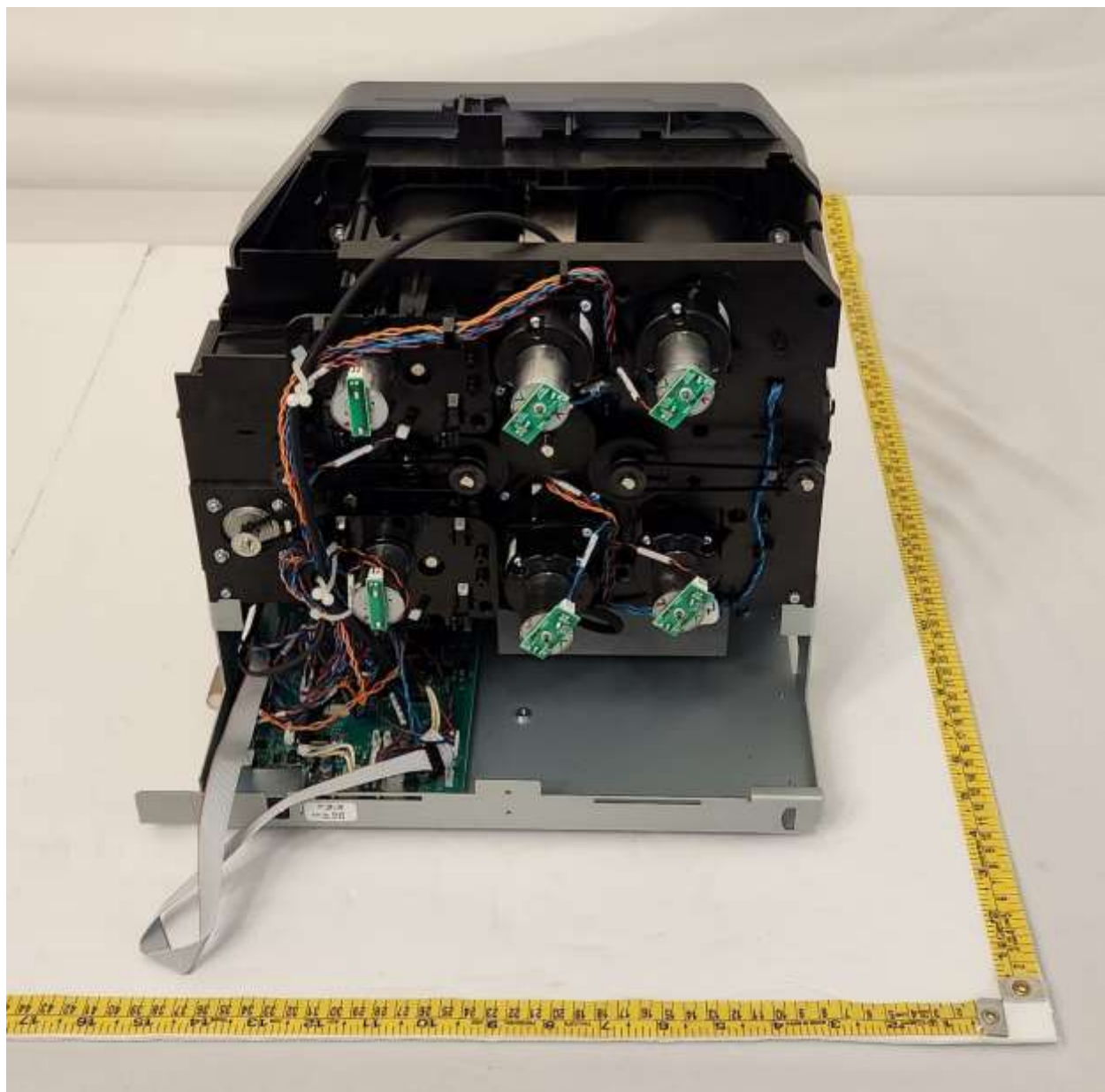
Laminator_Rear
