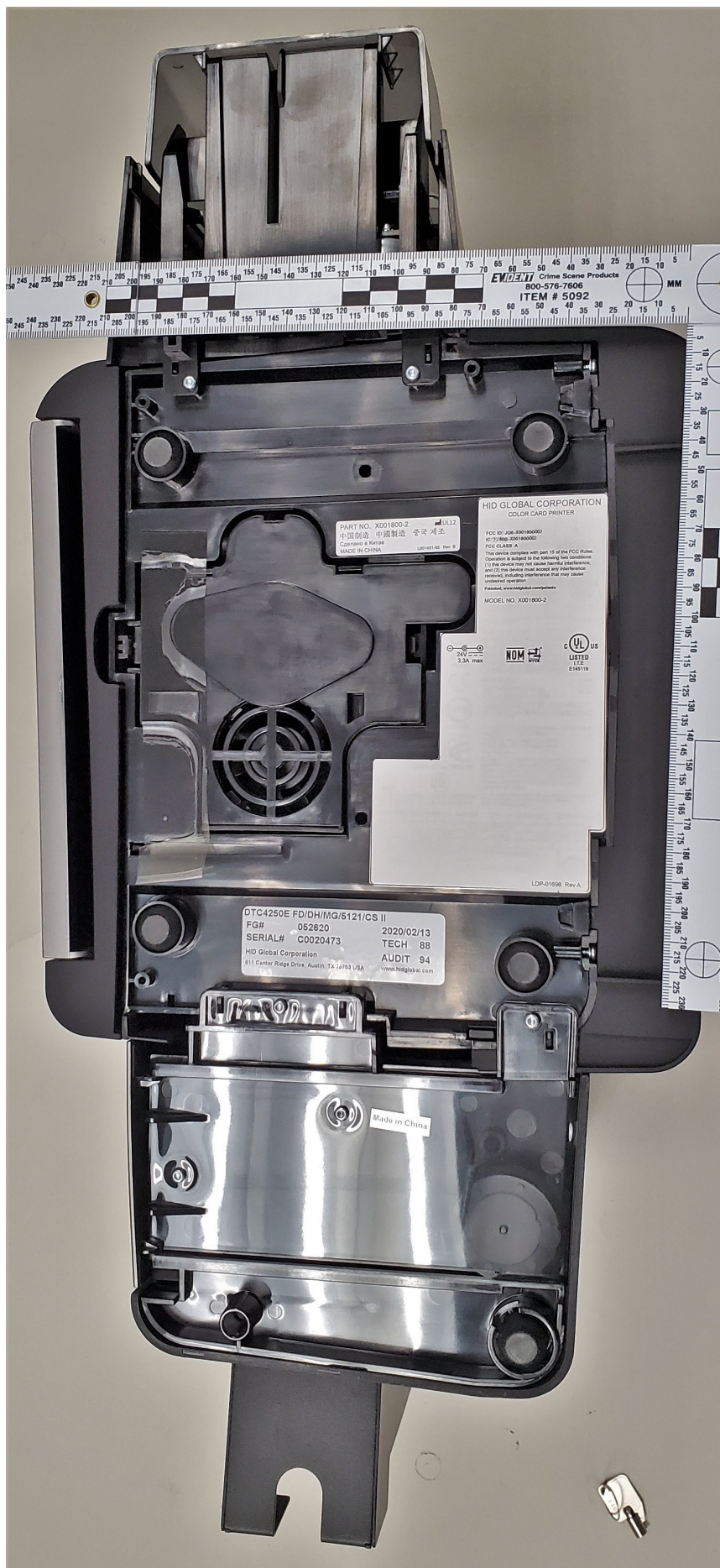
Bottom Side
