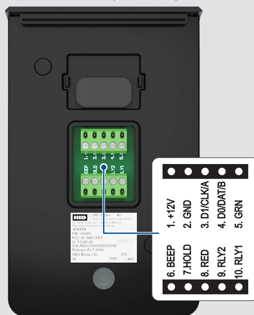
ターミナルストリップバージョン
