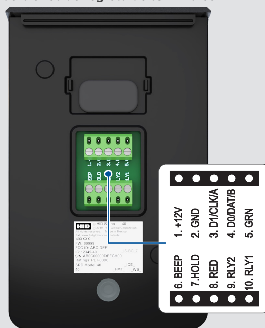
Versiones de regleta de terminales
