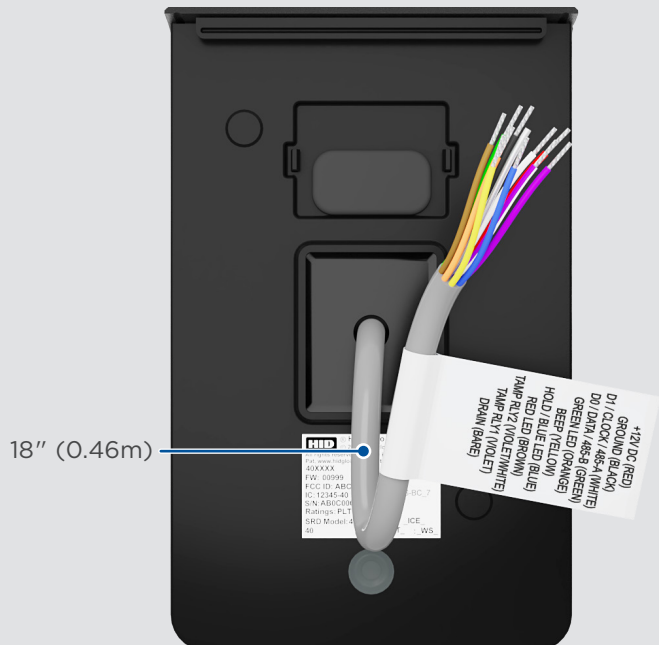
Versiones con cables flexibles
