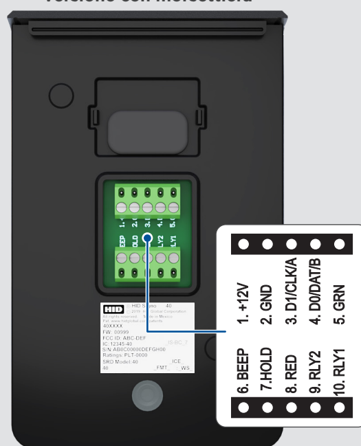
Versione con morsettiera
