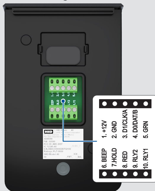
Versão com régua de bornes
