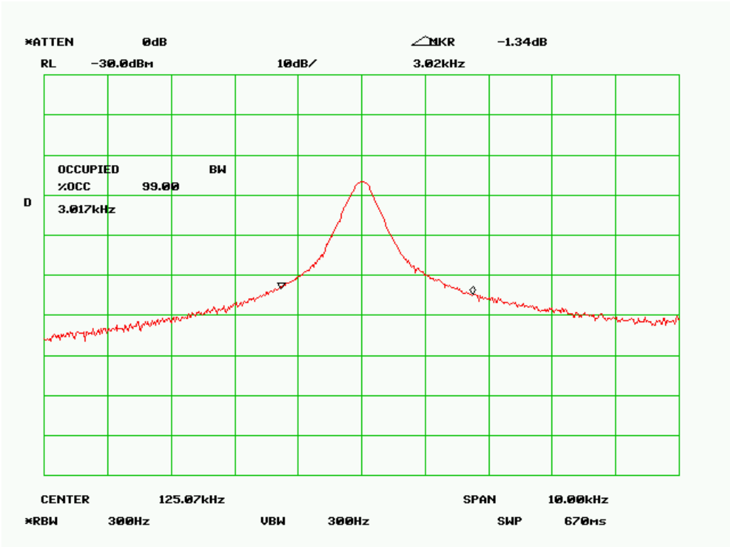
Plots: 125 kHz
