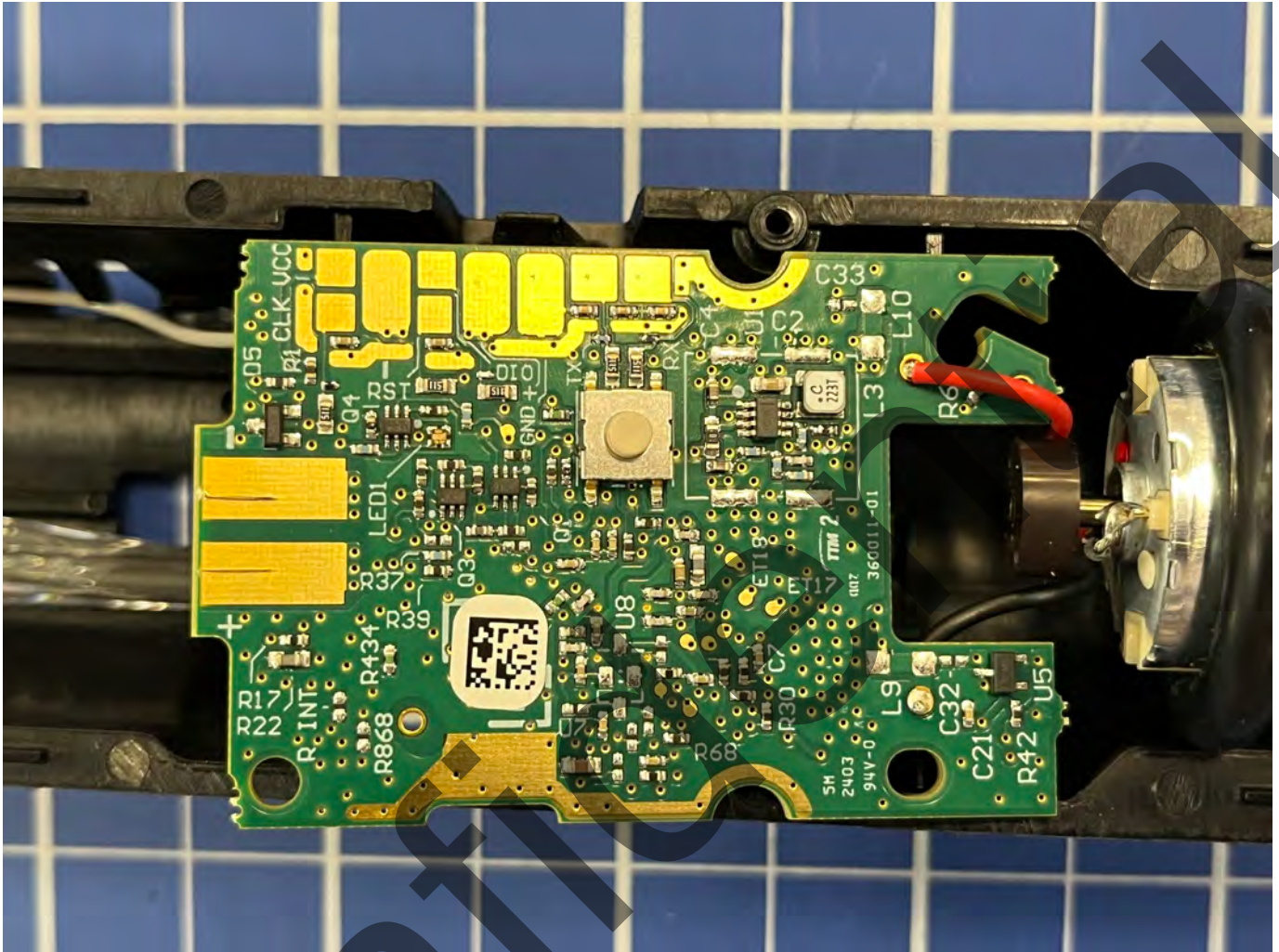
Bottom PCB
