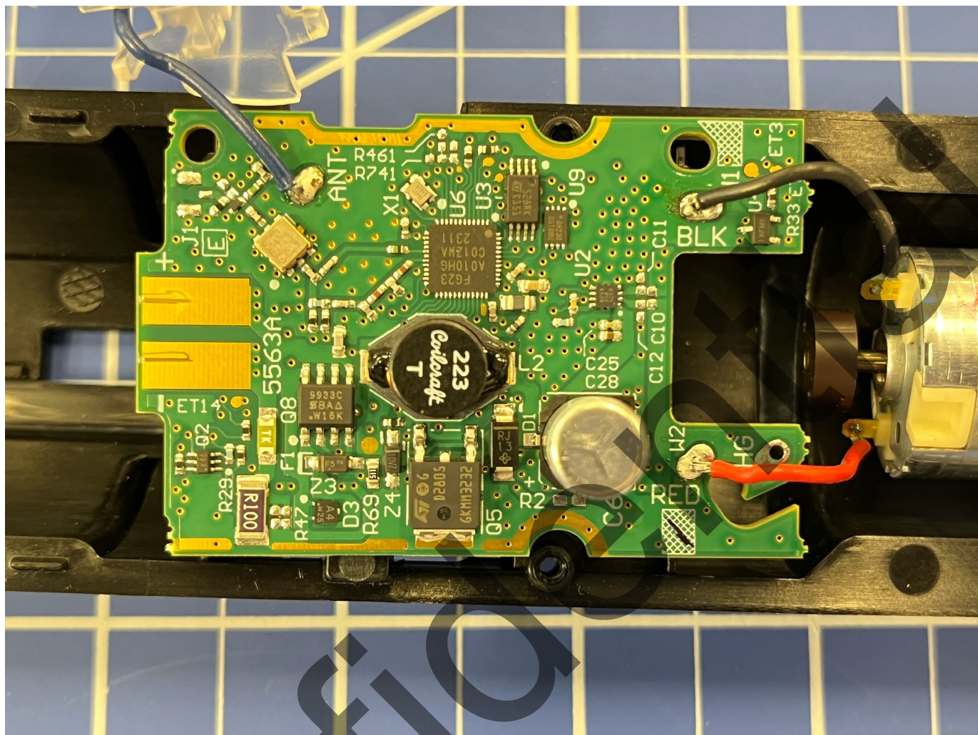
Top PCB
