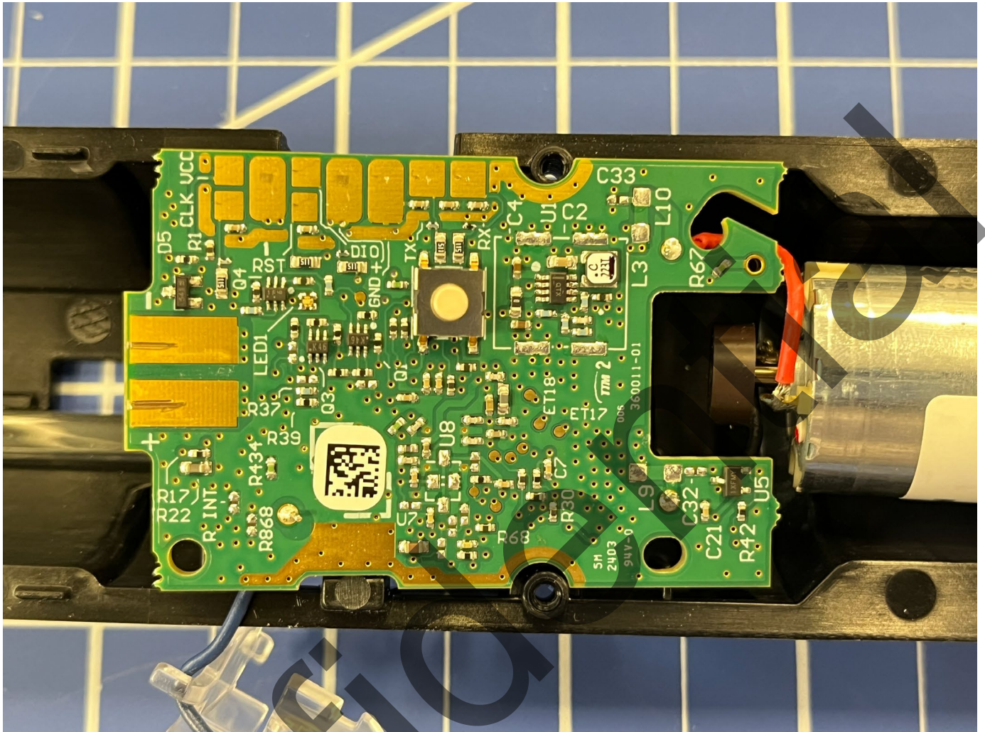
Bottom PCB
