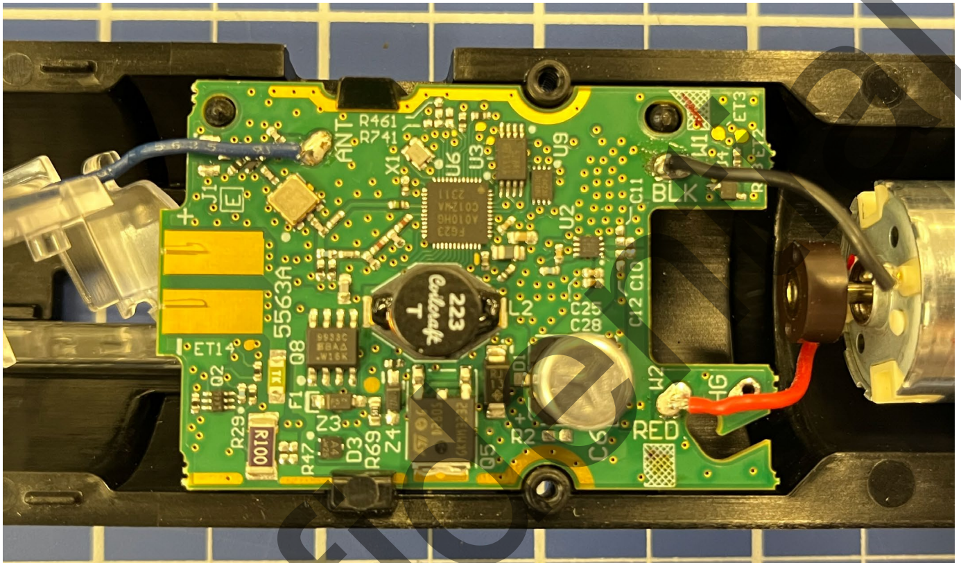
Top PCB
