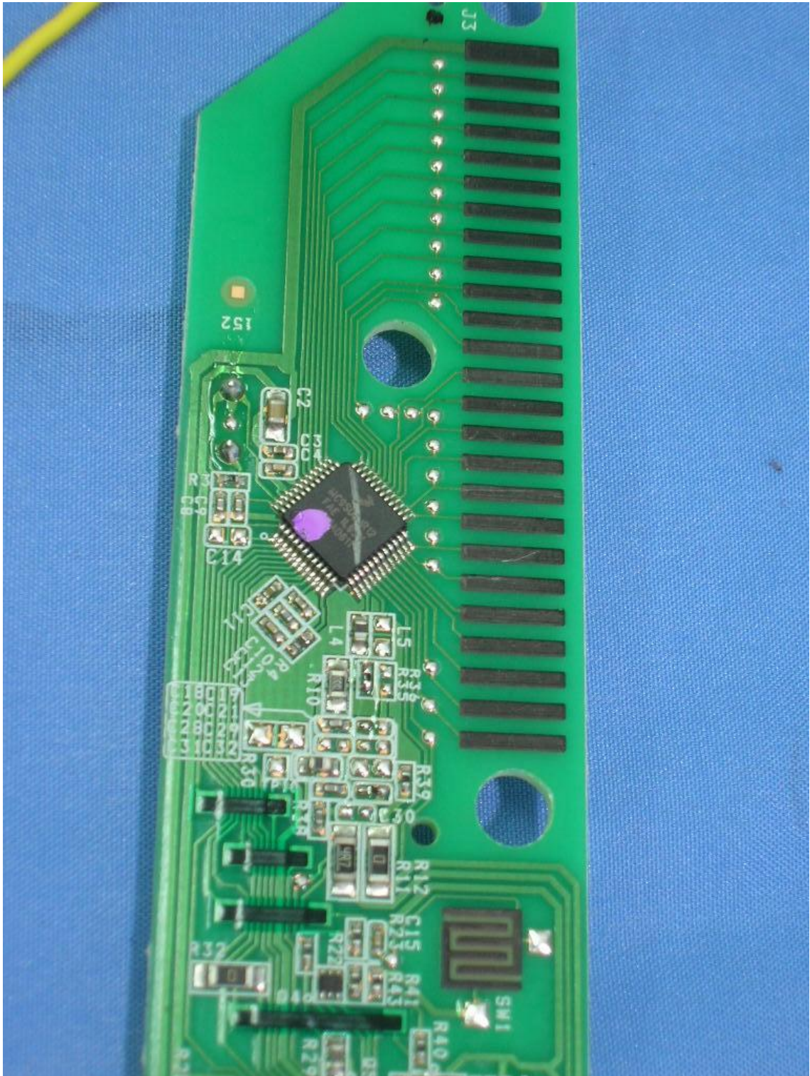
(12) EUT Photo
