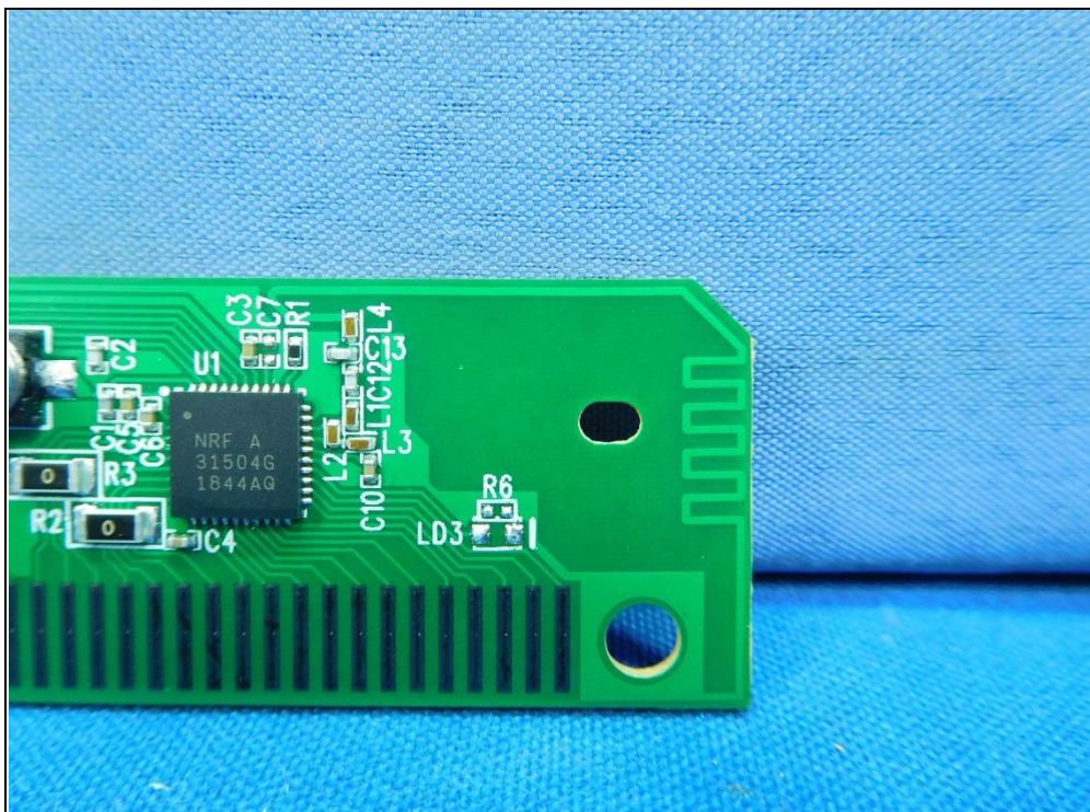
Antenna
