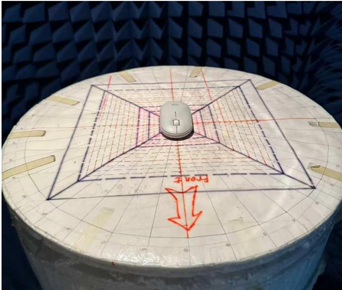
DUT plane 1
