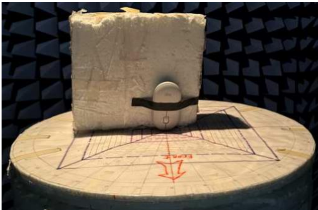
DUT plane 2
