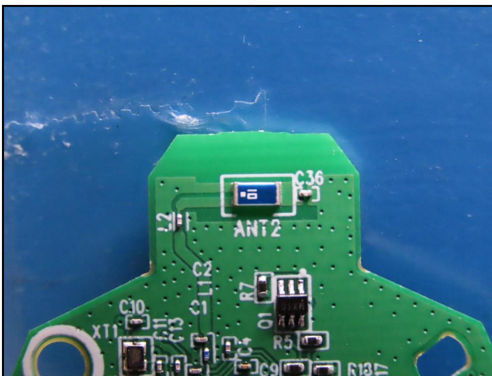
Antenna
