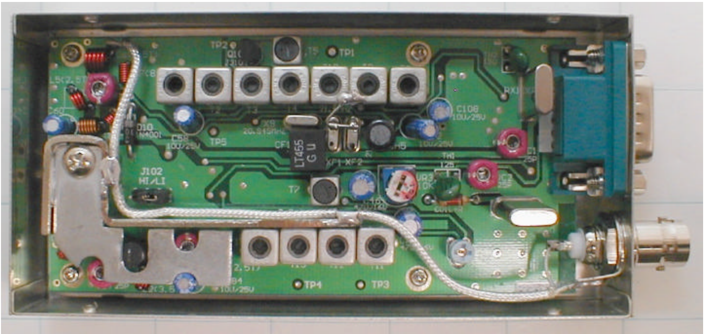
PCB Top
