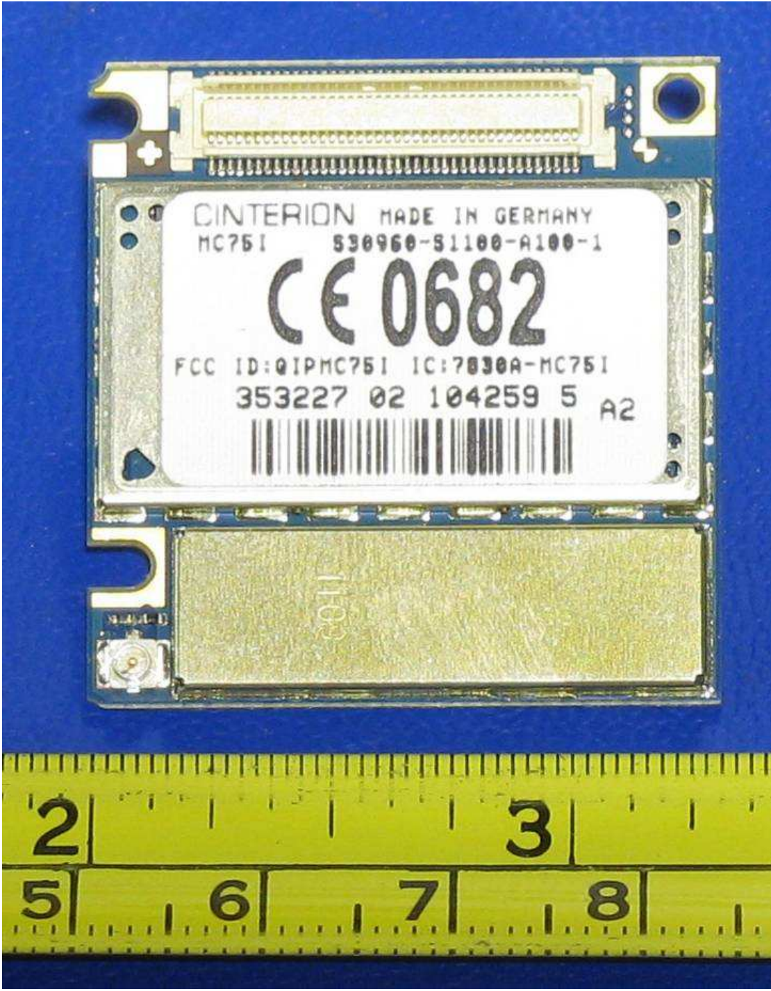
GSM Module
