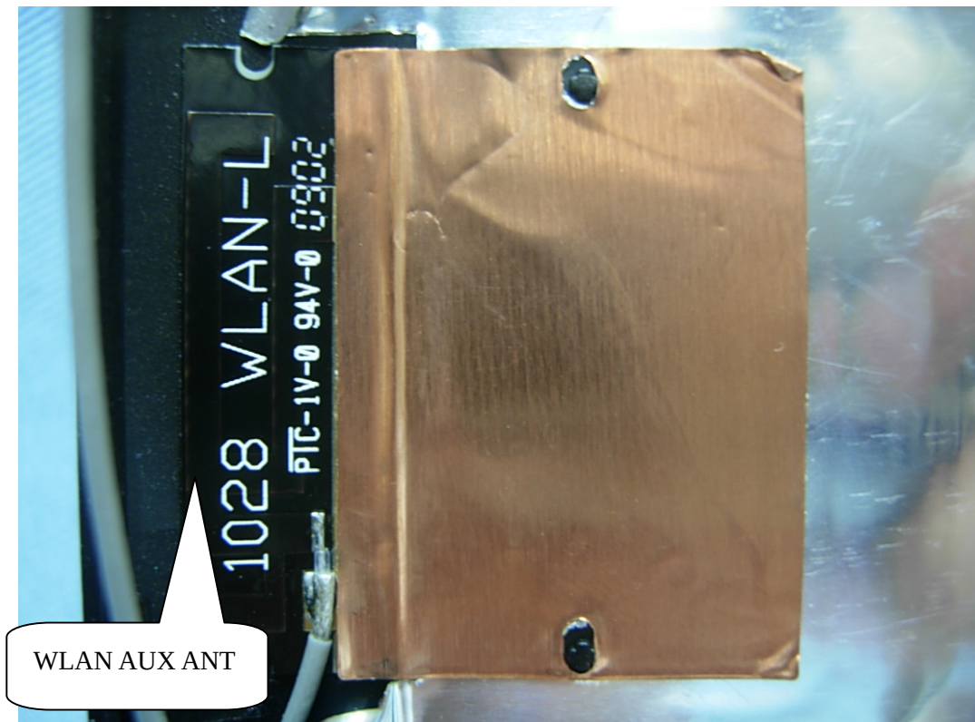
(8) EUT Photo
