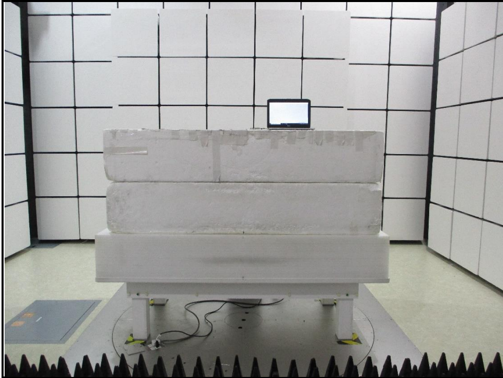
WiFi 6G , Eut X-Y
