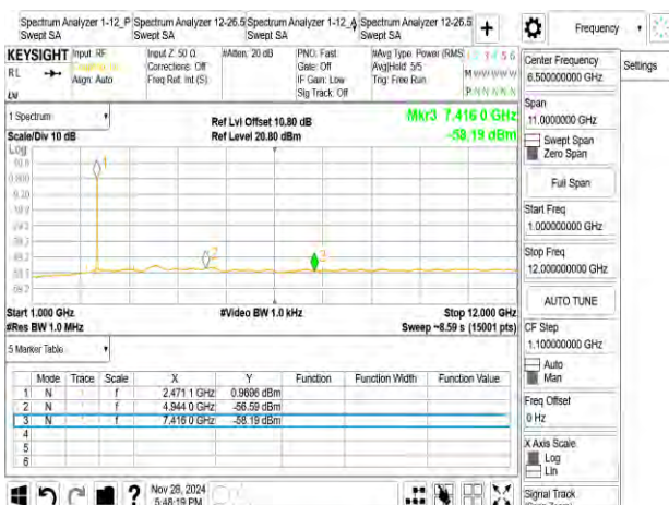
802_11b_20M_2472MHz
