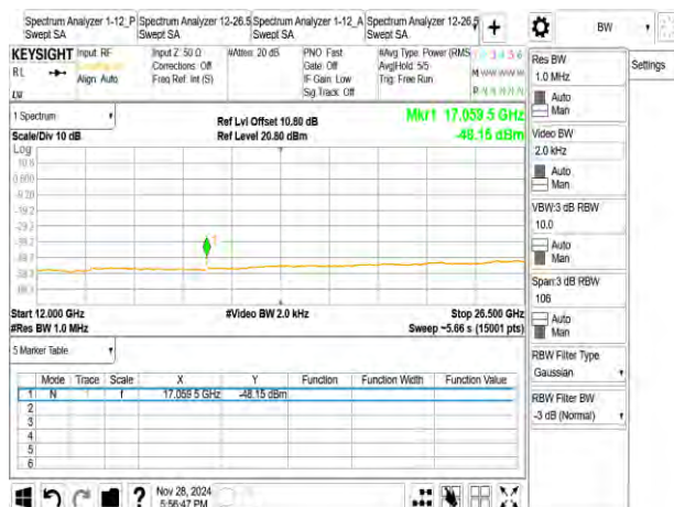
802_11g_20M_2462MHz
