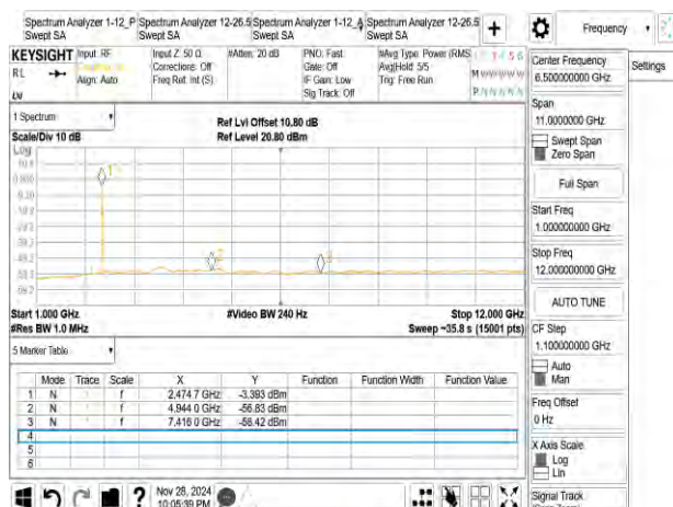
802_11ax_20M_2472MHz_RU106_54
