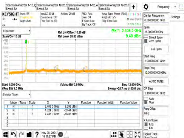
802_11ax_20M_2412MHz_RU242
