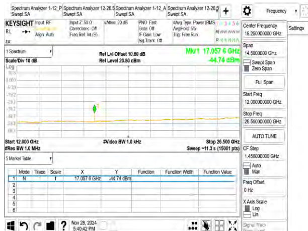
802_11b_20M_2462MHz
