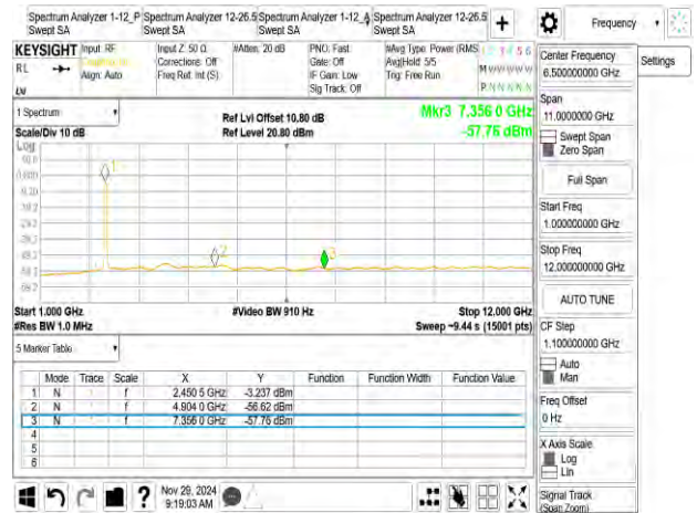
802_11ax_40M_2457MHz
