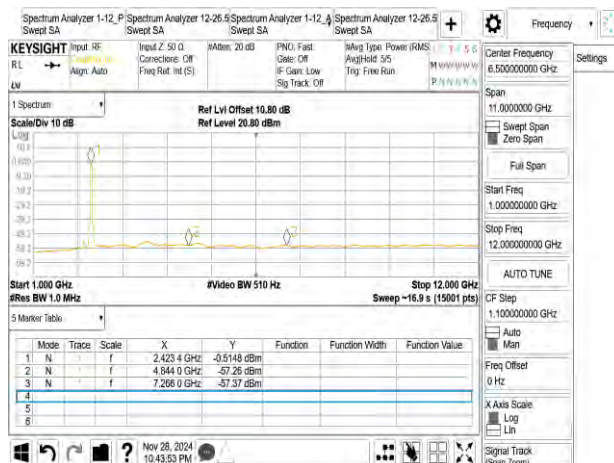
802_11ax_40M_2422MHz_RU242_61
