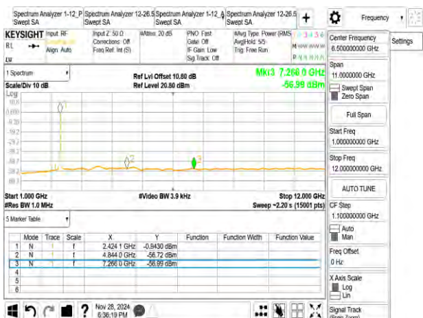
802_11n_40M_2437MHz
