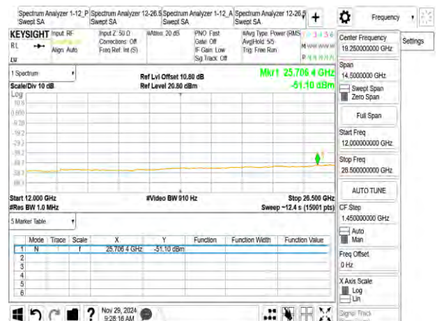
802_11ax_40M_2457MHz_RU484
