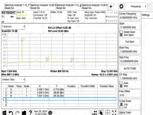
802_11ax_20M_2467MHz_RU242
