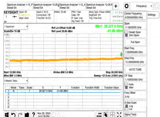
802_11g_20M_2467MHz
