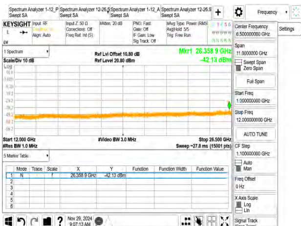
802_11ax_40M_2452MHz_RU484
