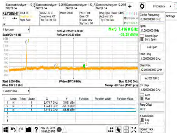
802_11ax_20M_2472MHz_RU106_54
