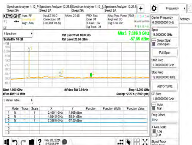
802_11n_40M_2462MHz
