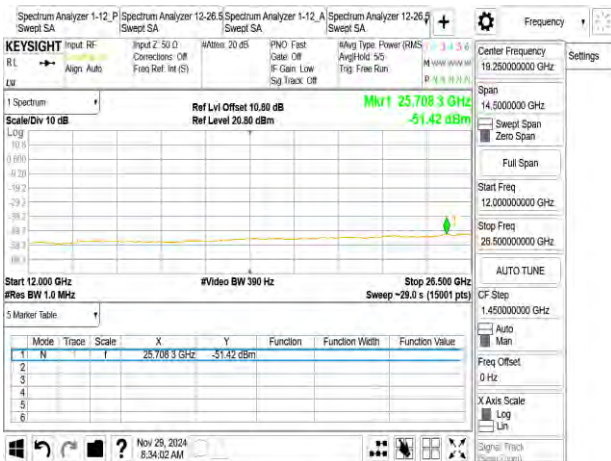
802_11ax_40M_2452MHz_RU484
