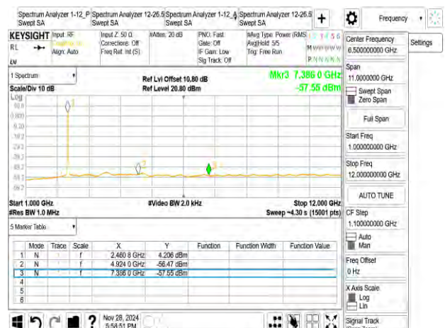
802_11g_20M_2462MHz
