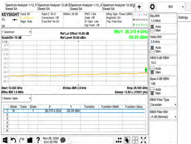
802_11n_40M_2452MHz
