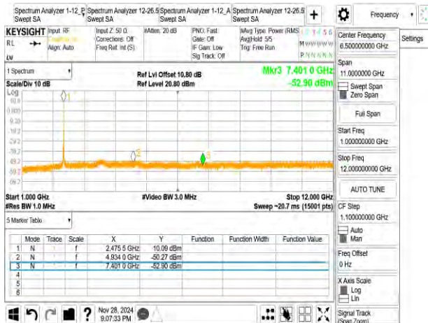
802_11ax_20M_2472MHz
