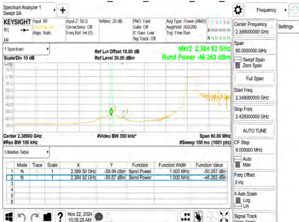
802.11ax_20MHz_2422MHz_RU52_37
