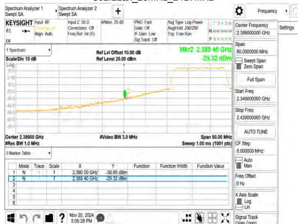
802.11ax_20MHz_2417MHz
