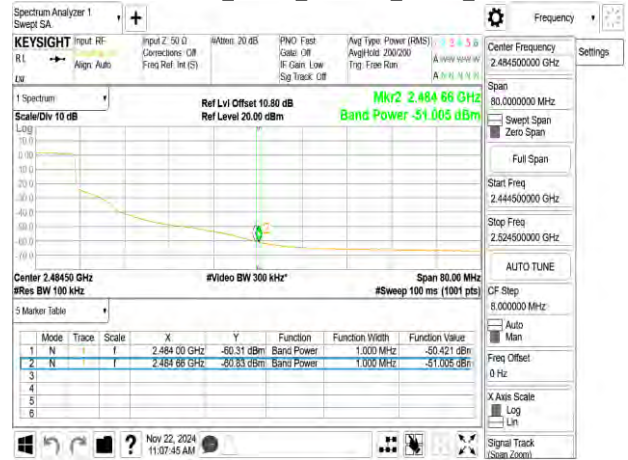
802.11ax_20MHz_2442MHz_RU242
