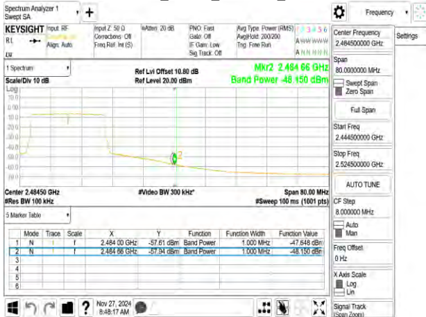
802.11ax_20MHz_2457MHz_RU26_8
