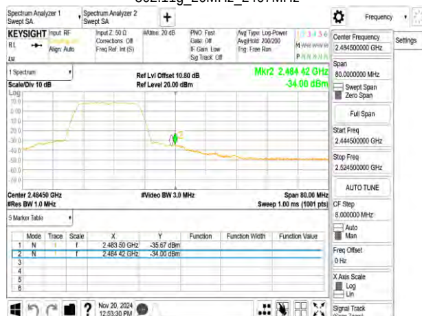
802.11g_20MHz_2472MHz
