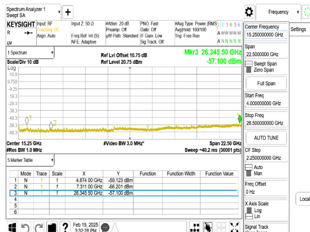
802.11ax_20MHz_Chain0_2437MHz_RU242_4-26.5GHz
