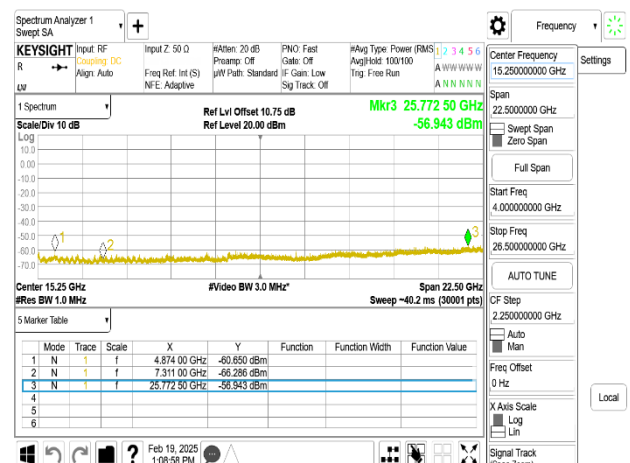
802.11n_20MHz_Chain0_2437MHz_4-26.5GHz
