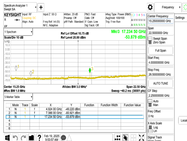
802.11b_20MHz_Chain0_2462MHz_4-26.5GHz
