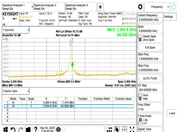
802.11n_40MHz_Chain0_2462MHz_1-4GHz
