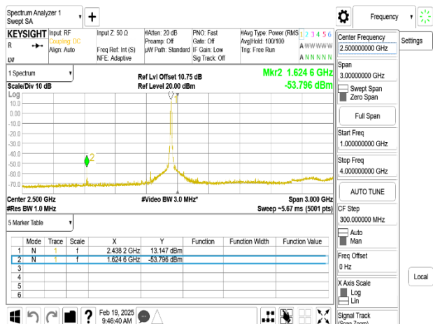
802.11b_20MHz_Chain0_2437MHz_1-4GHz
