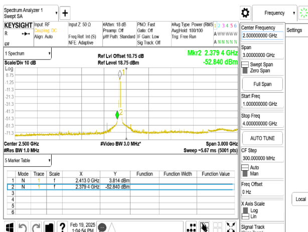
802.11n_20MHz_Chain0_2412MHz_1-4GHz
