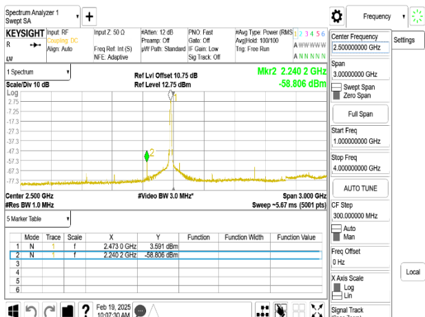
802.11b_20MHz_Chain0_2472MHz_1-4GHz
